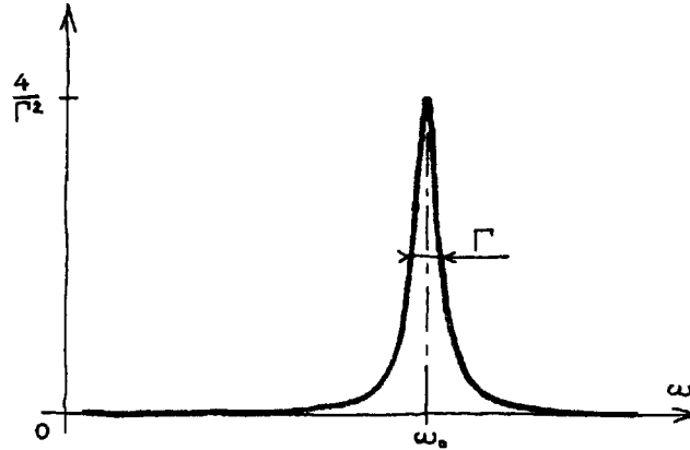
Figure VI.4: Le graphe de la lorentzienne \frac{1}{(\omega - \omega_0)^2 + \frac{1}{4}\Gamma^2} .
