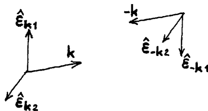
Figure III.2: Un choix de vecteurs polarisation de base du mode -\mathbf{k} .
