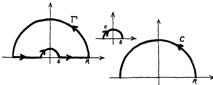
Figure II.5: Les contours d'intégration pour évaluer \int_{-\infty}^{\infty} dz \frac{1-e^{iz}}{z^2} .
