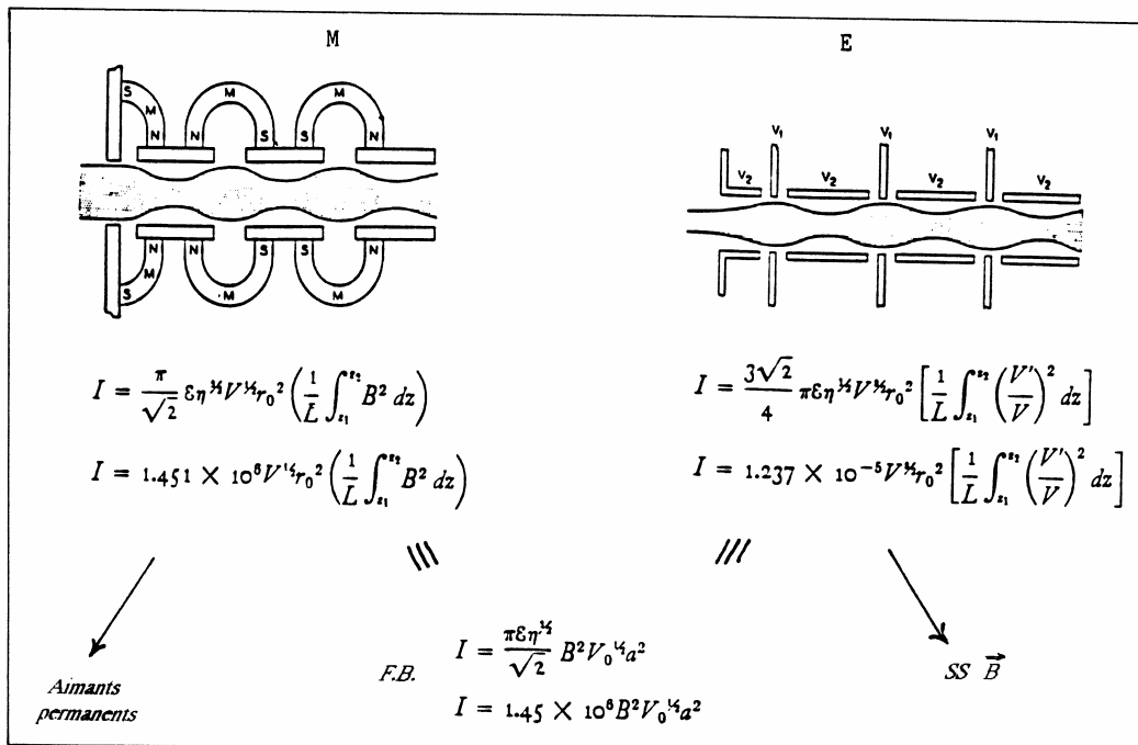
Figure XII-3-3 - Focalisations périodiques.
