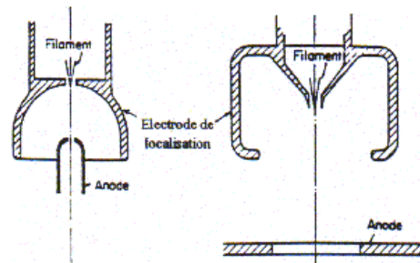
Figure III-2-7 - Exemples de canon haute brillance
