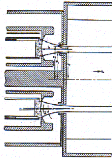
b) Canon magnétron extérieur.
