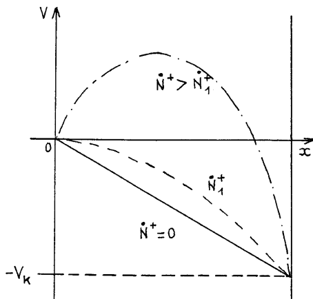
Figure VII-3-2 - Variations de potentiel A-K dans un plasma.
