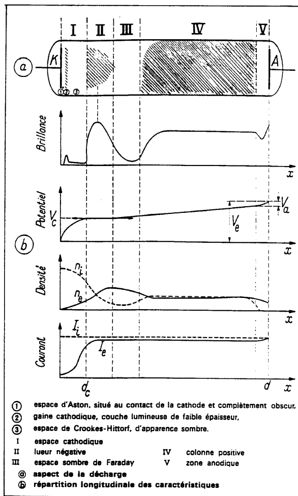
Figure VII-5-4 - Caractéristiques d'une décharge lumineuse basse pression.
