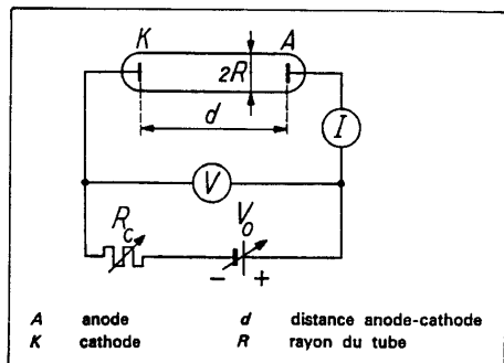
Figure VII-5-1 - Schéma d'un tube de décharge.
