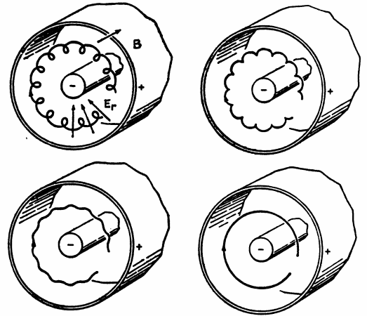
Figure I-1-6 - Mouvements magnétron.
