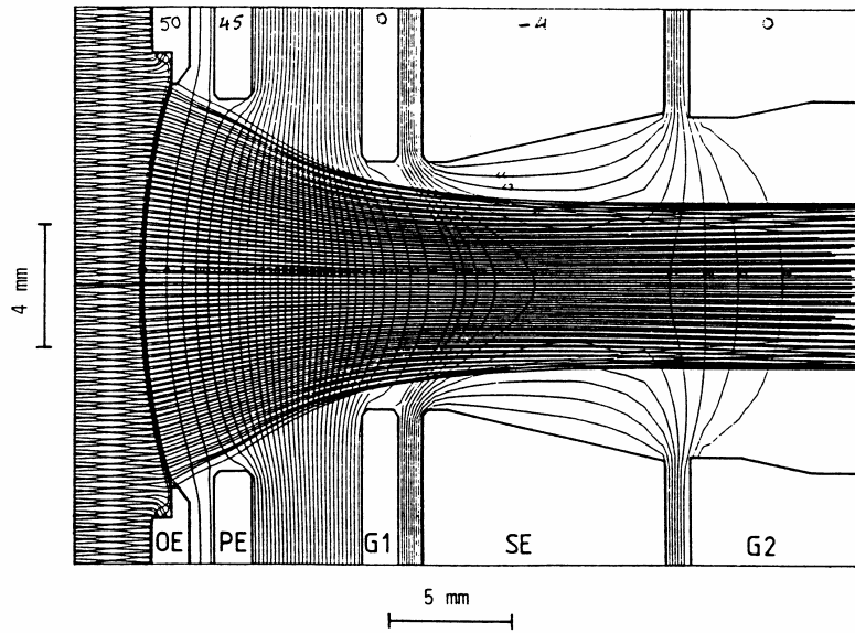
Figure XII-5-7 - Calcul self-consistent d'une extraction ionique (AXCEL).
