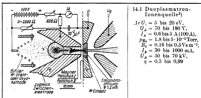
Figure VIII-1-3a - Duoplasmatron.
