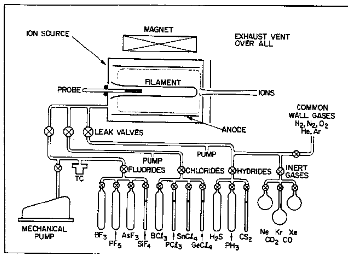
Figure V-3-1 - Schéma d'un système d'injection de gaz.
