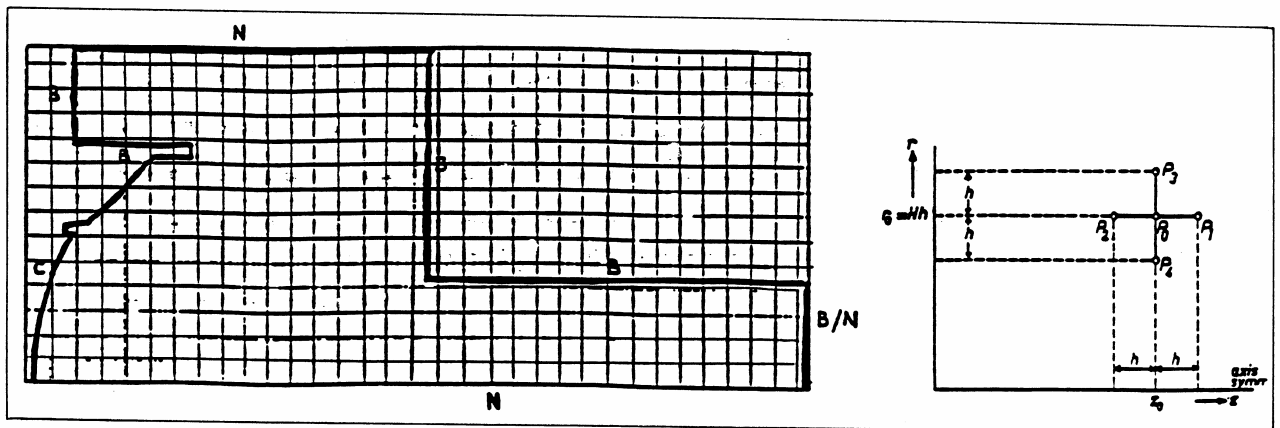
Figure XII-4-2 - Maillage carré.
