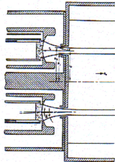
b) Canon magnétron extérieur.
