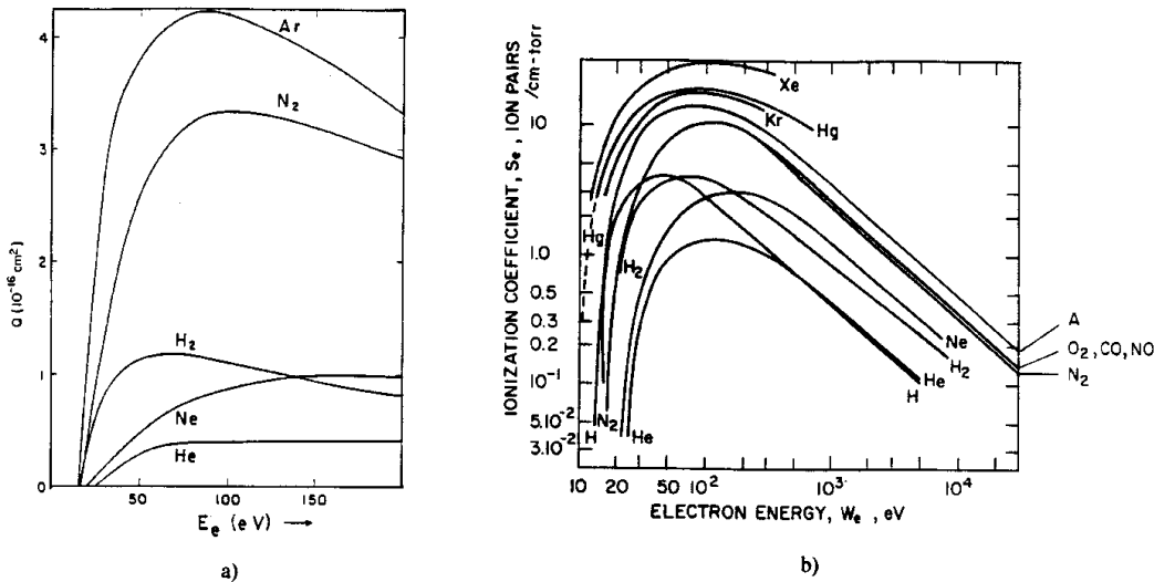
Figure VI-1-3 - Variation de la section efficace de première ionisation.
