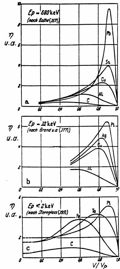
Figure II-4-9 - Distribution des $e^-$ rétrodiffusés.
