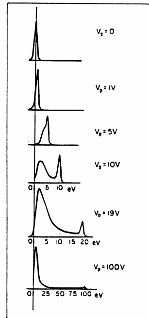
Figure II-4-8 - Distribution des électrons secondaires à basse énergie incidente.
