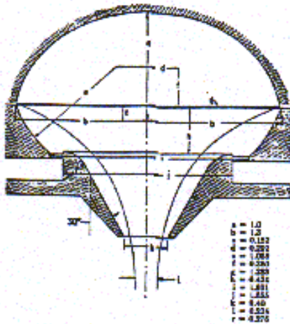
a) Canon de Heil.
