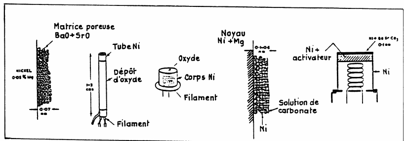
Figure II-1-22 - Cathodes à oxydes.
