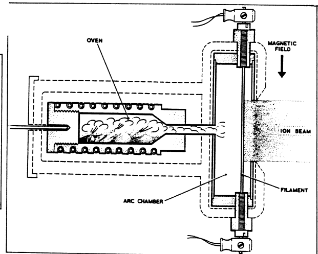
Figure VIII-1-11a - Schéma de la source Freeman.
