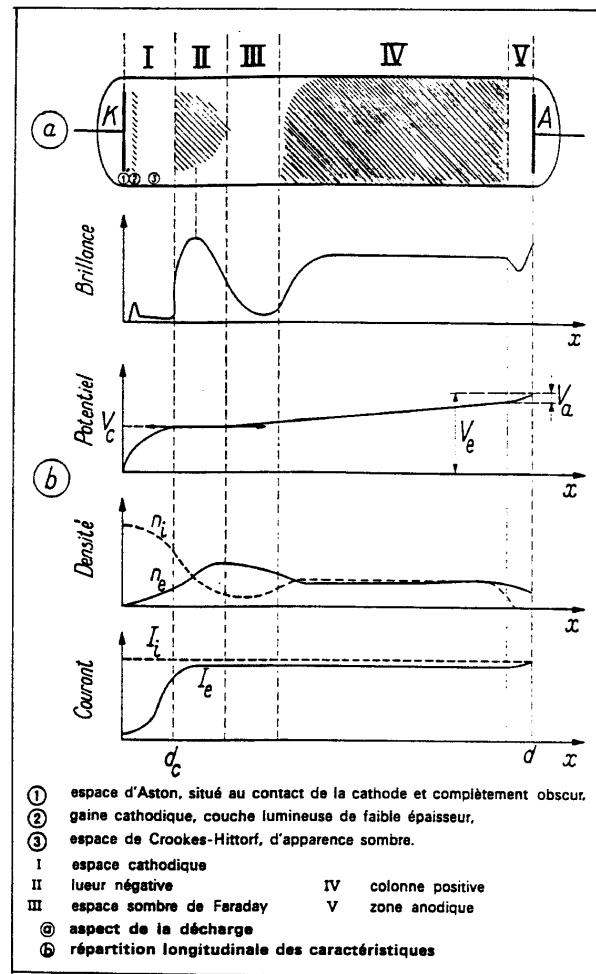
Figure VII-5-4 - Caractéristiques d'une décharge luminescente basse pression.
