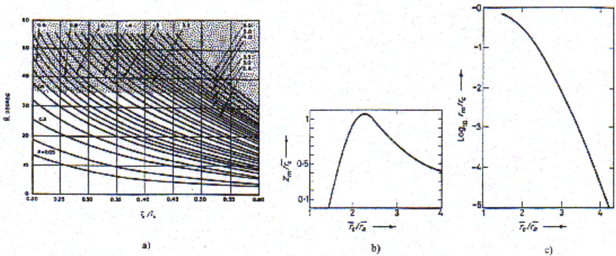
Figure III-1-3 - Graphes de mise au point d'un canon de Pierce.
