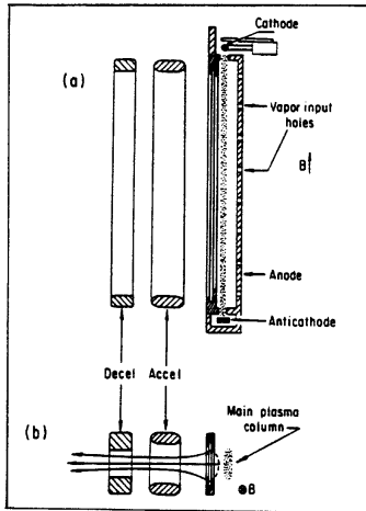
Figure VIII-1-9 - Calutron.
