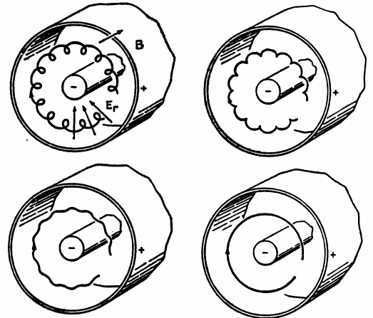
Figure I-1-6 - Mouvements magnétron.
