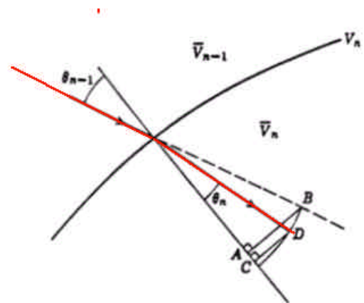
Figure XII-6-8 - Loi de Descartes en électrostatique.
