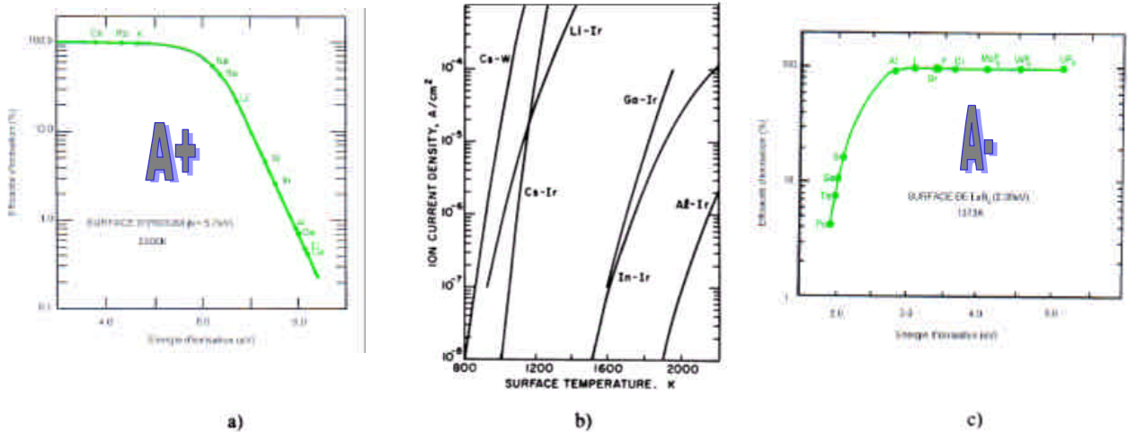
Figure VI-2-1 - Variations des efficacités d'ionisation de surface \eta et \gamma avec I , A et \phi .
