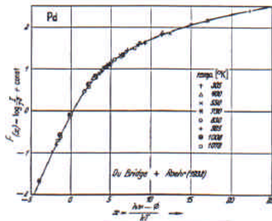
Figure II-3-1 - Photoémission de Pd à 8 températures.
