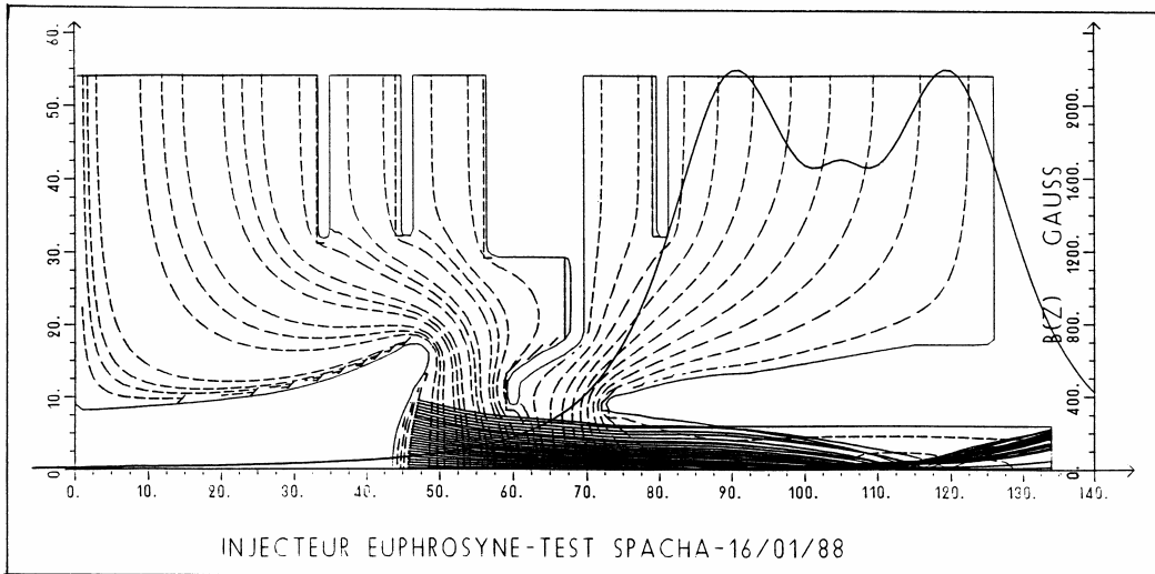
Figure XII-4-1a - Exemple de simulation numérique (EGUN).
