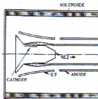
c) Canon magnétron immergé.
