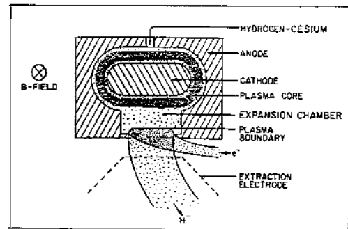
Figure IX-2-2 - Source magnétron.
