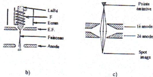
Figure III-2-7 - Exemples de canon haute brillance
