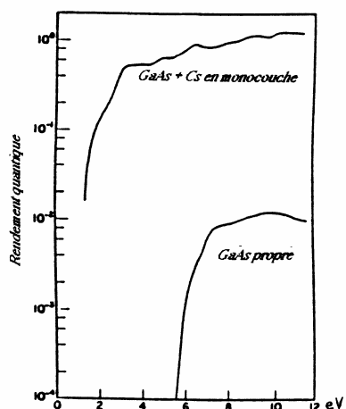
Figure II-3-4 - Rendement quantique de GaAs.
