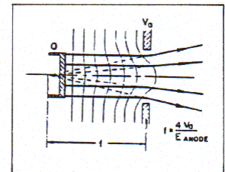
Figure III-1-5 - Effet de l'ouverture anodique.
