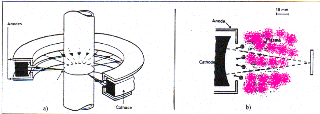
Figure III-1-10 - Canon à plasma pour raffinage.
