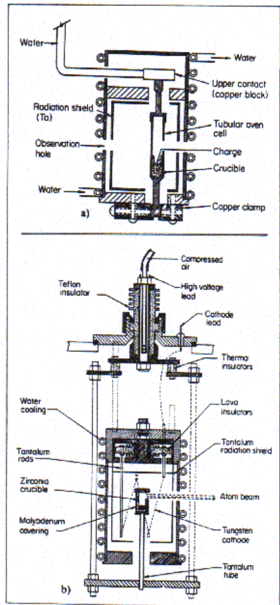
Figure V-2-5 - Fours haute température.
