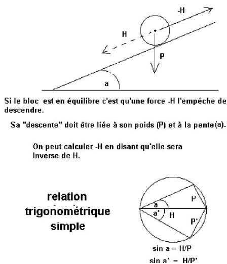
Figure 1 : équilibre théorique sur une pente.
