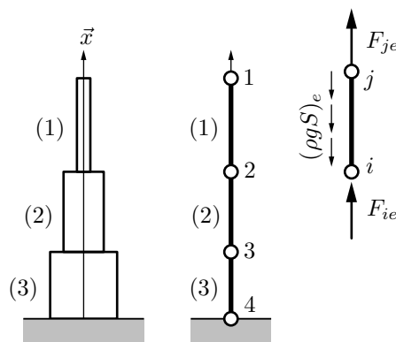
Figure A.9 - Colonne et efforts élémentaires
