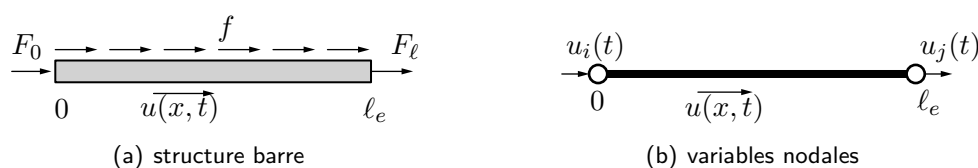
Figure 3.1 - Modèle barre
