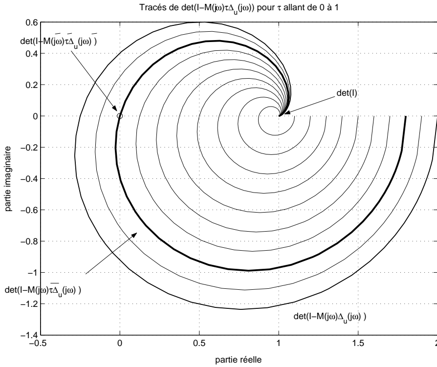
FIG. 3.19 – Tracés de \det(I - M(j\omega)\tau\Delta_u(j\omega)) , \omega allant de 0 à +\infty , pour \tau allant de 0 à 1
