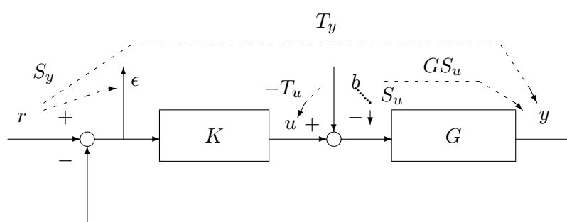
FIG. 9.1 – Système en boucle fermée MIMO
