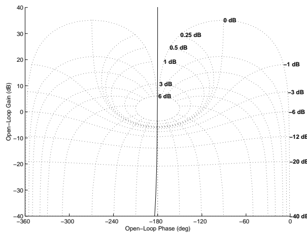
FIG. 5.8 – Diagramme de Nichols de \frac{k^c}{j\omega} G(j\omega) avec k^c = 0,01
