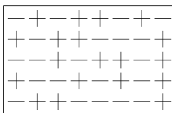
FIGURE 3.4. Une configuration du modèle d'Ising en dimension d = 2 .
