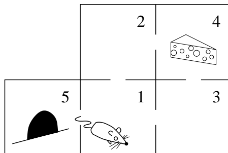
FIGURE 3.1. Le labyrinthe dans lequel vit la souris.
