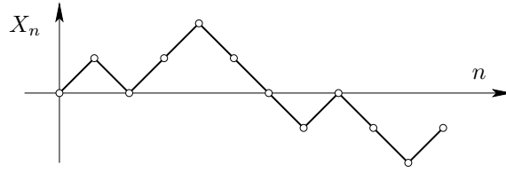
FIGURE 4.2. Une réalisation d'une marche aléatoire unidimensionnelle.
