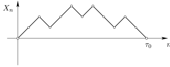
FIGURE 4.3. Une réalisation d'une marche aléatoire unidimensionnelle pour laquelle \tau_0 = 12 .
