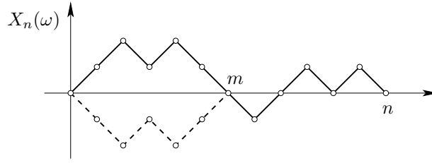
FIGURE 4.4. Pour chaque réalisation d'une marche aléatoire avec \tau_0 = m < n telle que X_1 = 1 , il existe une autre réalisation telle que \tau_0 = m et X_1 = -1 , obtenue par réflexion par rapport à l'axe des abscisses.
