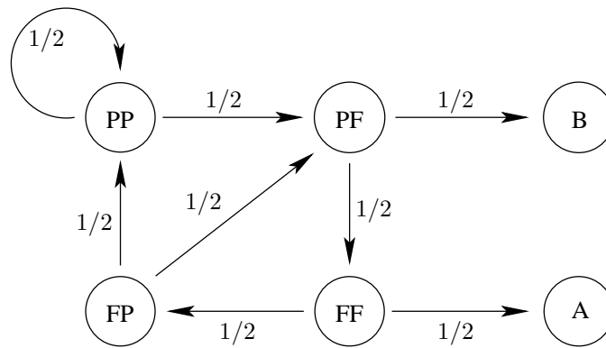
FIGURE 3.2. Graphe associé au jeu de Pile ou Face. Chaque symbole de deux lettres représente le résultat des deux derniers jets de pièce. Anatole gagne si la pièce tombe trois fois de suite sur Face, Barnabé gagne si la pièce tombe sur Pile-Face-Pile.
