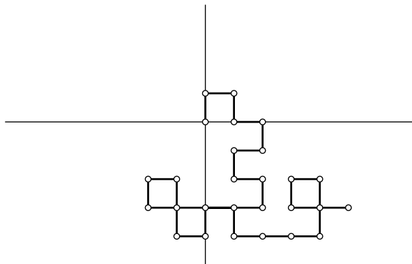
FIGURE 4.1. Une trajectoire d'une marche aléatoire en dimension d = 2 .
