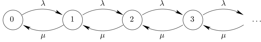
FIGURE 7.1. Graphe associé à la file d'attente M/M/1.
