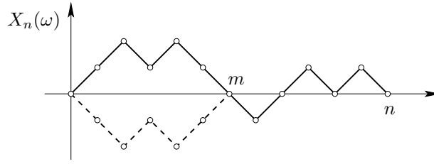
FIGURE 2.4. Pour chaque réalisation d'une marche aléatoire avec \tau_0 = m < n telle que X_1 = 1 , il existe une autre réalisation telle que \tau_0 = m et X_1 = -1 , obtenue par réflexion par rapport à l'axe des abscisses.
