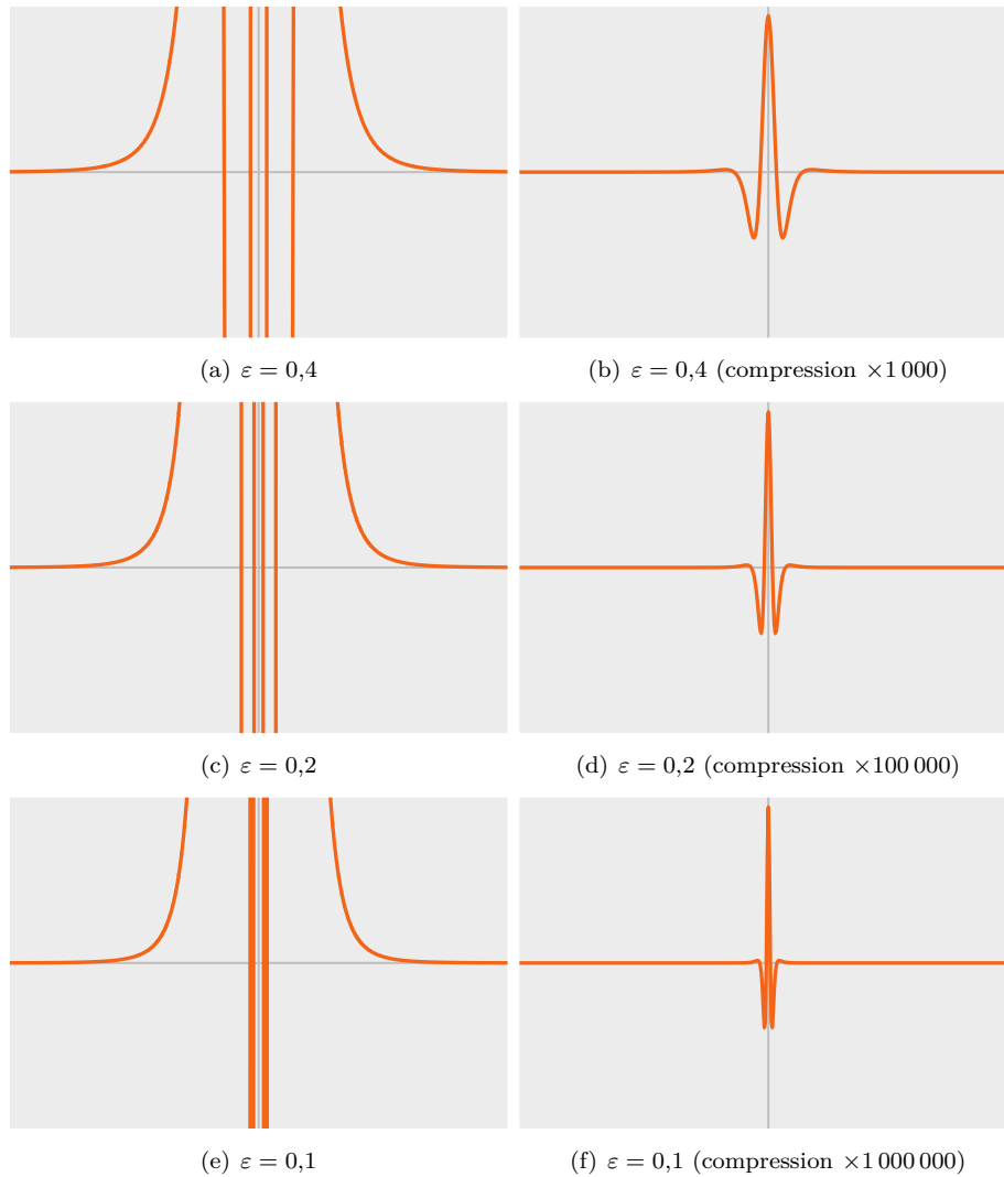
Figure VIII.6 – Compression de la fonction I_{-4,\epsilon} — À gauche, les deux maxima latéraux sortent du champ; les portions de courbe qui vont d'un extremum au suivant n'apparaissent plus que comme des droites verticales. À droite, l'ordonnée est comprimée pour ramener les extrema dans le champ, ce qui rend invisibles les maxima latéraux
