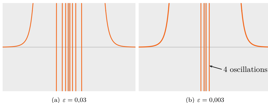
Figure VIII.7 – Fonctions I_{-8; \varepsilon}(x) — Le nombre d'oscillations a doublé par rapport au cas précédent. Les extrema sont énormes : de l'ordre de 10^{18} pour \varepsilon = 0,03 et de 10^{27} pour \varepsilon = 0,003 .
