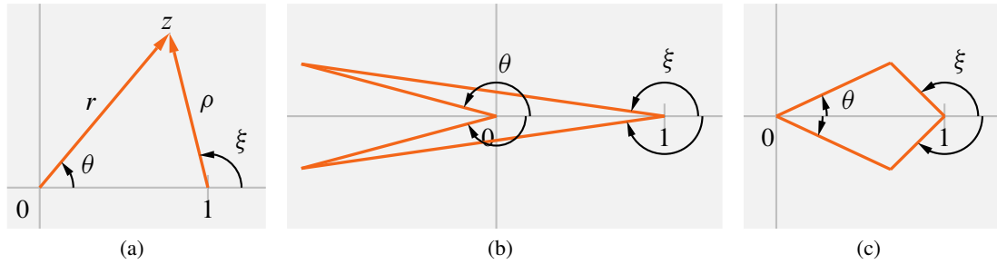
Figure IV.9 — Passage à la limite dans les expressions [z^\alpha]_1 \cdot [(z - 1)^\beta]_1
