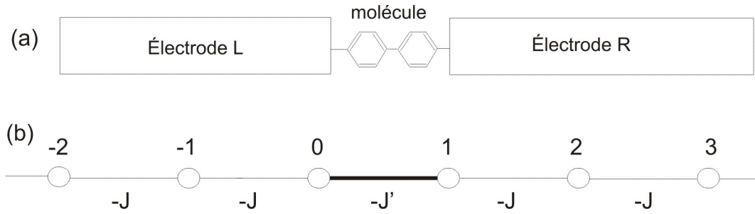
FIGURE 8.2 – Modélisation de la jonction métal-molécule-métal
