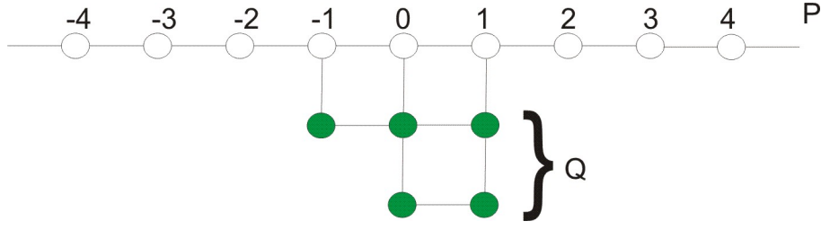
FIGURE 3.4 – Réseau perturbé par un cluster attaché sur les sites -1,0 et 1.
