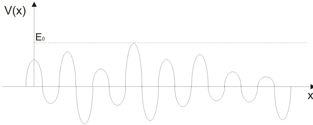
FIGURE 6.1 – Mouvement d’une particule dans un réseau 1D aléatoire.
