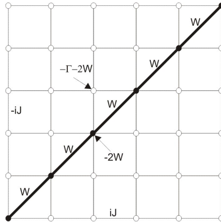
FIGURE 7.1 – Représentation de l'espace de Liouville 2D
