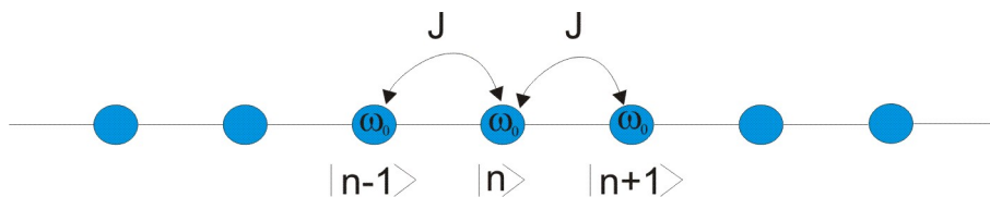
FIGURE 2.1 – Représentation du réseau
