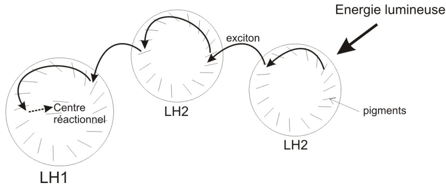
FIGURE 1.2 – Schéma des complexes LH1 et LH2 collectant l'énergie lumineuse et la transférant sous forme excitonique au centre réactionnel.
