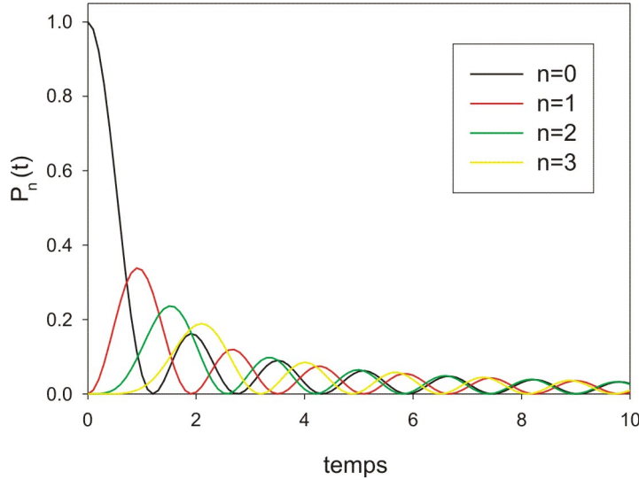
FIGURE 2.3 – Evolution temporelle de la densité d'énergie en unité Jt .
