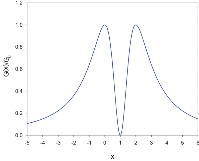
FIGURE 5.6 – Variation de la conductance de la jonction en fonction x = (J - J')/J .
