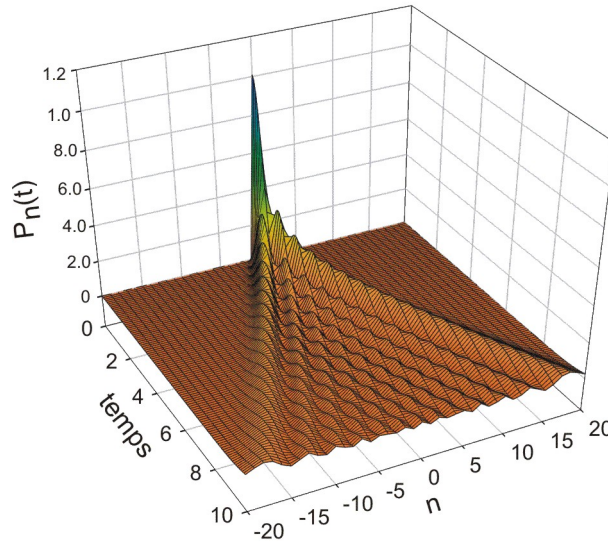
FIGURE 2.4 – Evolution spatio-temporelle de la densité d'énergie en unité Jt .
