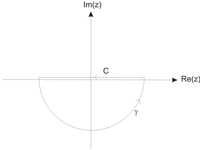
FIGURE 2.2 – Contours C et \gamma dans le plan complexe.
