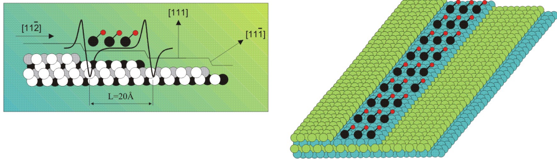
FIGURE 1.4 – Confinement de molécules sur une surface vicinale de platine.
