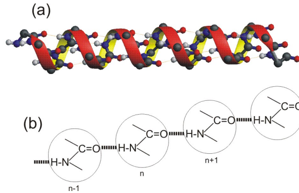
FIGURE 1.1 – (a) Représentation 3D d’une hélice- \alpha . (b) Sous réseau particulier d’unités peptidiques connectées par les liaisons hydrogènes.
