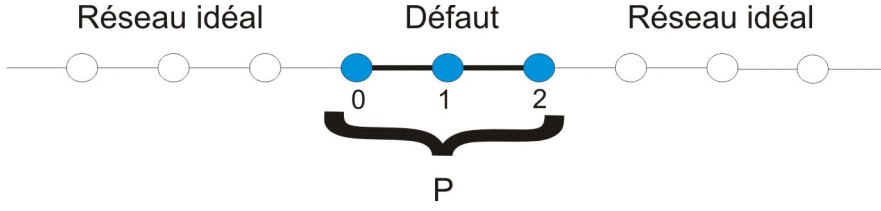
FIGURE 3.1 – Réseau présentant un défaut de petite taille affectant les sites 0,1 et 2.
