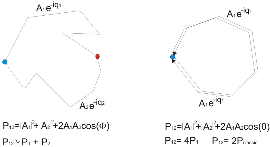
FIGURE 6.2 – Contribution de deux chemins à la probabilité de transition entre deux sites.
