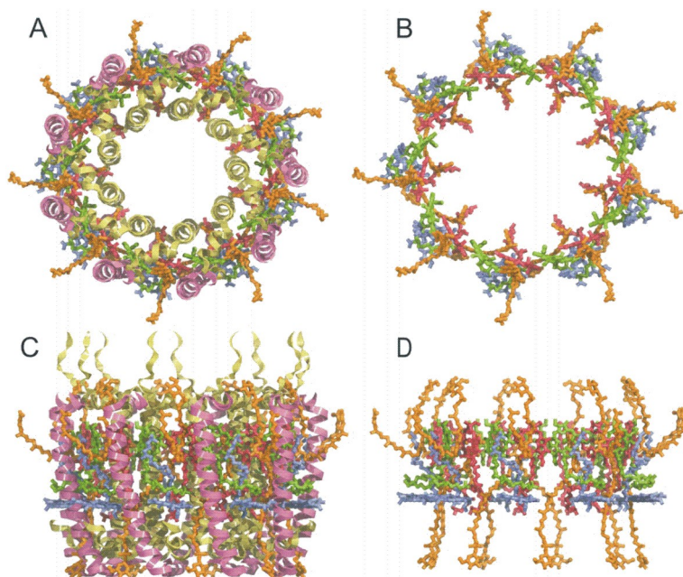
FIGURE 1.3 – Représentation du complexe LH2 : vue dans la surface de la membrane (a) et (b) ; vue le long de la surface de la membrane (c) et (d).
