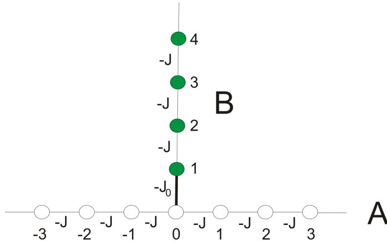
FIGURE 8.4 – Modèle de deux réseaux orthogonaux interconnectés
