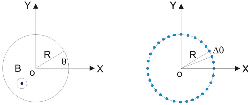
FIGURE 5.4 – Modèle des liaisons fortes pour un anneau traversé par le flux d'un champ magnétique
