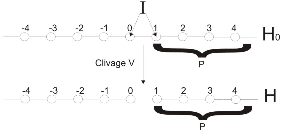
FIGURE 3.3 – Clivage du réseau idéal pour former deux réseaux indépendants.
