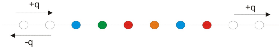
FIGURE 6.2 – Contribution de deux chemins à la probabilité de transition entre deux sites.
