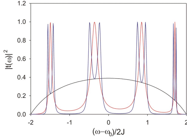
FIGURE 4.1 – Transmittance à travers un (noir), deux (rouge) et trois (bleu) défauts séparés de L = 5 sites pour \Delta/J = 2.5
