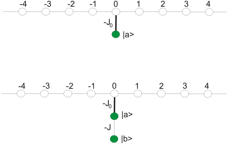
FIGURE 8.1 – Modélisation d'un cluster attaché à un nano-fil.
