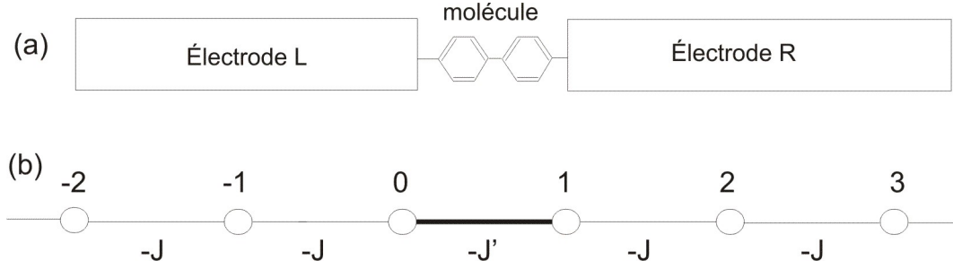
FIGURE 5.5 – Modélisation de la jonction métal-molécule-métal.
