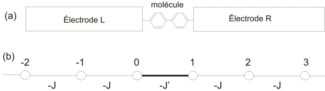
FIGURE 8.2 – Modélisation de la jonction métal-molécule-métal
