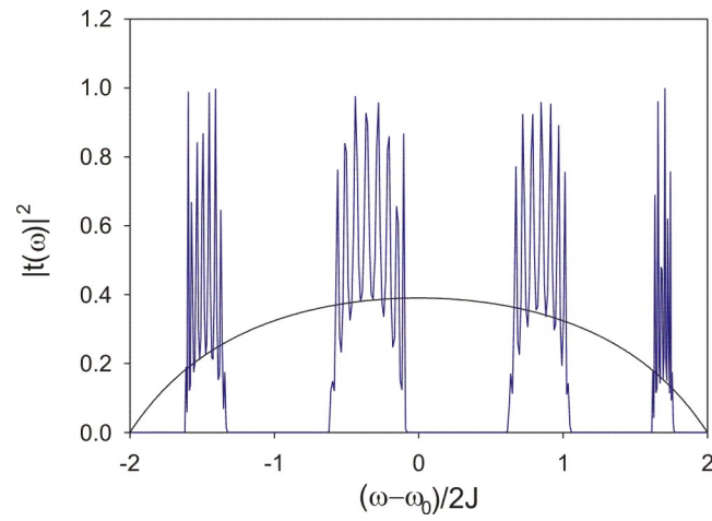
FIGURE 4.2 – Transmittance à travers un (noir) et dix (bleu) défauts séparés de L = 5 sites pour \Delta/J = 2.5
