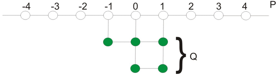
FIGURE 3.4 – Réseau perturbé par un cluster attaché sur les sites -1,0 et 1.
