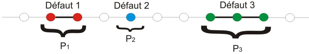
FIGURE 3.2 – Réseau présentant un ensemble de défauts.
