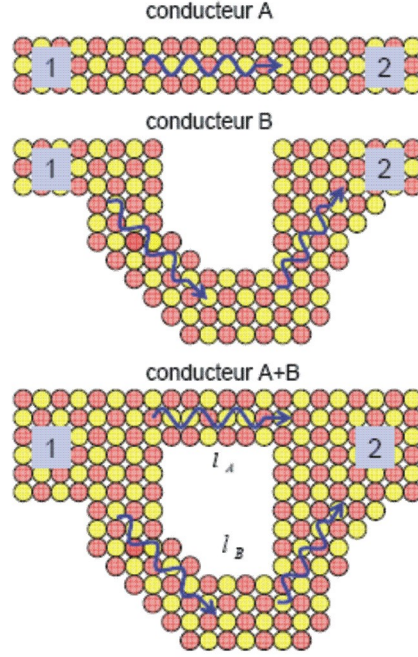
FIGURE 5.2 – Conductance de deux conducteurs quantiques en parallèle.
