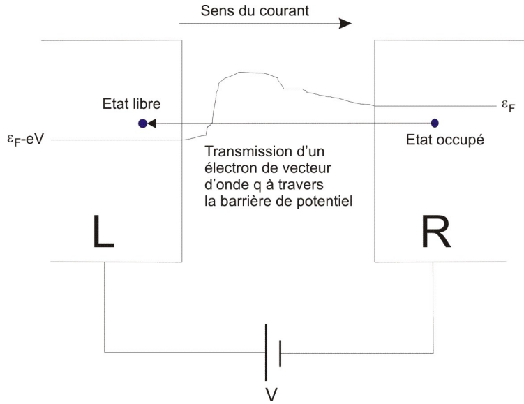
FIGURE 5.1 – Courant entre deux conducteurs quantiques.
