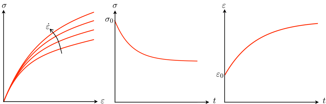
FIGURE 2.7 – Mise en évidence d’un comportement avec viscosité : à gauche, dépendance de la réponse à la vitesse de déformation ; au milieu, relaxation de la contrainte à déformation constante ; à droite, fluage à contrainte constante.
