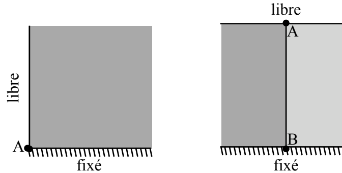
FIGURE 5.2 – Exemple de points singuliers en élasticité plane : à gauche, le point A à l'angle droit d'un changement de type de conditions aux limites ; à droite, les points A et B , à l'interface de deux matériaux et sur un bord libre ou un bord fixé. De tels points ne seraient pas singuliers en élasticité anti-plane.
