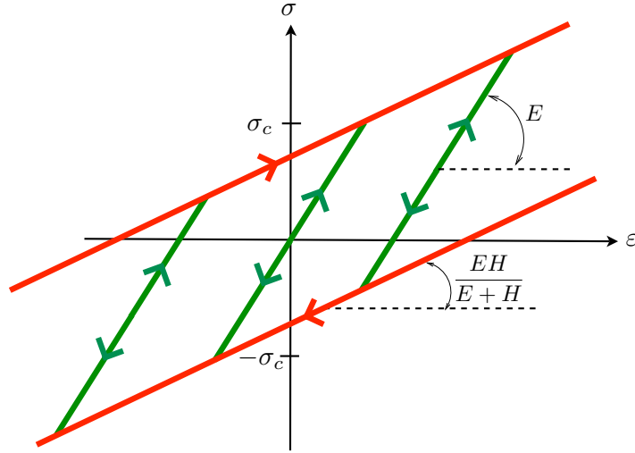
FIGURE 3.9 – Diagramme résumant le comportement de l'assemblage ressort-patin-ressort. En rouge : les phases irréversibles de glissement du patin ; en vert : les phases réversibles de blocage du patin.
