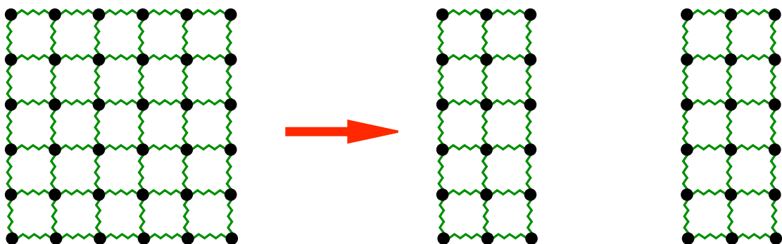
FIGURE 6.6 – Séparation en deux blocs d'un réseau d'atomes et justification de l'énergie de fissuration. (Les ressorts symbolisent les interactions entre plus proches voisins.)
