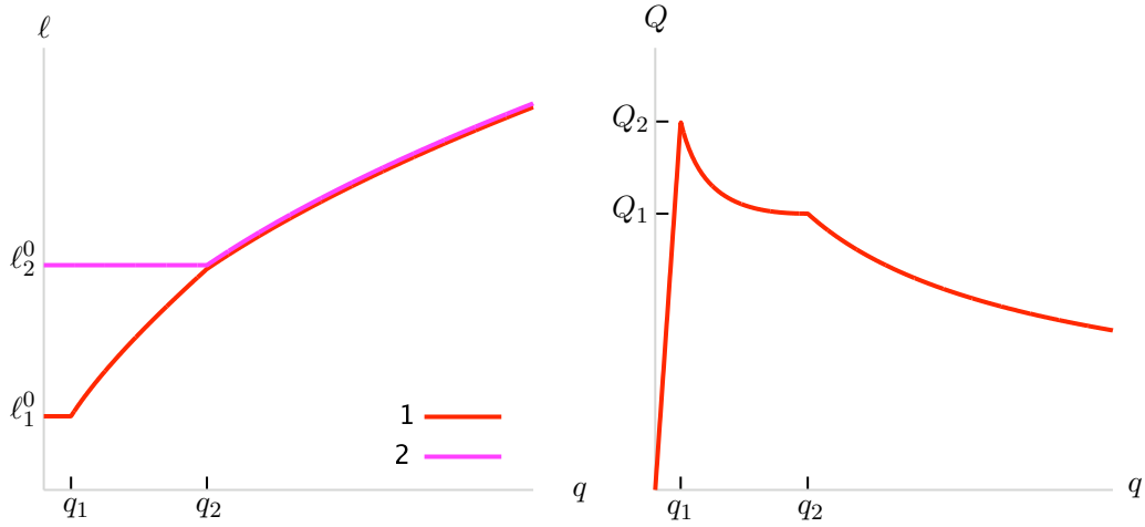
FIGURE 7.3 – Solution du problème de décollement d’un revêtement. À gauche, évolution des deux fronts en fonction du déplacement imposé ; à droite, évolution de la force associée en fonction du déplacement imposé.
