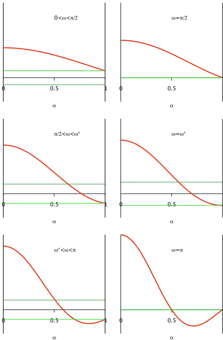
FIGURE 5.4 – Détermination graphique de la puissance de la singularité pour différentes valeurs de l'angle d'entaille. En rouge : le graphe de \alpha \mapsto \sin 2\alpha\omega/\alpha ; en vert clair : \sin 2\omega ; en vert foncé : -\sin 2\omega .
