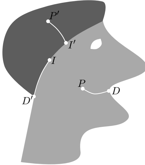
FIGURE 5.10 – Domaine bidimensionnel contenant trois fissures dont une d’interface et deux débouchantes au bord. Seules les pointes P et P' ont des singularités du type de celles étudiées dans cette section. Les points D , D' qui sont débouchantes et les points I et I' qui sont sur une interface relèvent d’études spécifiques.
