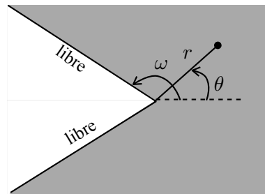
FIGURE 5.3 – Entaille d'angle 2\pi - 2\omega à bords libres.
