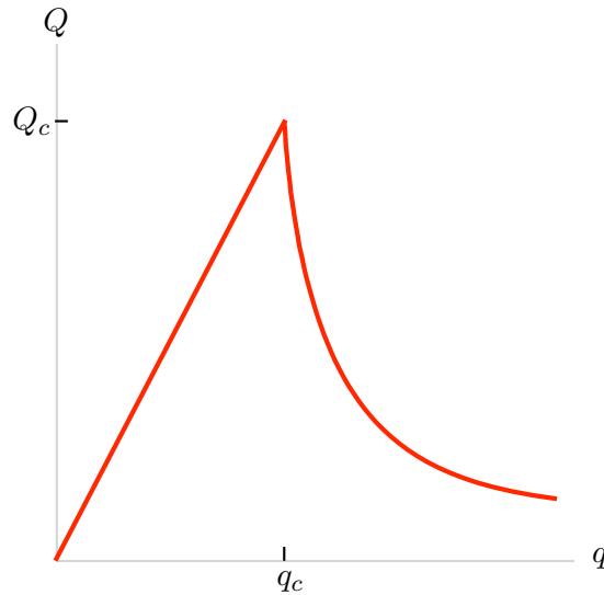
FIGURE 7.6 – Réponse de la poutre sous déplacement contrôlé croissant dans un diagramme force-déplacement prédite par la loi de Griffith. À noter le fort adoucissement.
