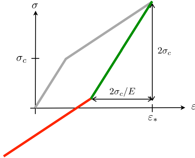
FIGURE 3.8 – Réponse de l’assemblage ressort-patin-ressort lors de la décharge. En vert : phase de blocage du patin ; en rouge : phase de glissement du patin vers la gauche.
