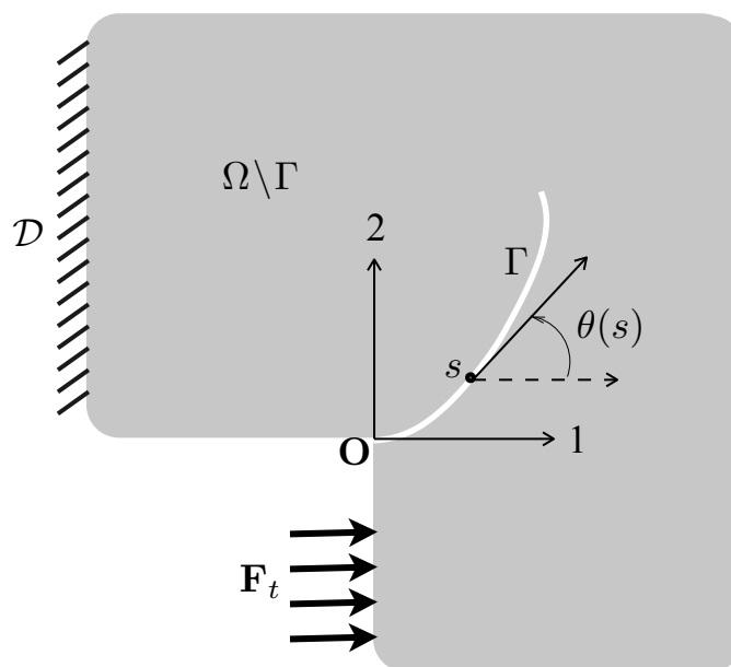
FIGURE 7.8 – Trajet d'une fissure en élasticité plane.
