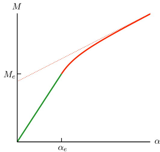
FIGURE 4.7 – Réponse globale de l'arbre plein sous torsion dans le cas d'un écroûssage cinématique linéaire.
