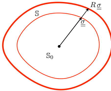
FIGURE 3.14 – Ecrouissage isotrope : dilatation du domaine de réversibilité.
