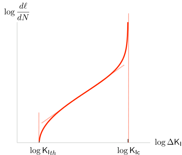
FIGURE 7.15 – Courbe expérimentale typique obtenue dans un essai de fatigue sous chargement cyclique
