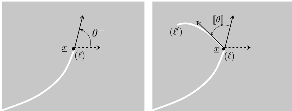
FIGURE 7.9 – Branchement d'une fissure en élasticité plane.
