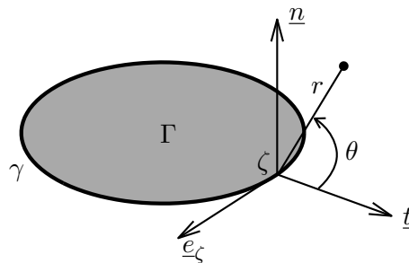
FIGURE 5.13 – Fissure en 3D : \Gamma est la surface de discontinuité, \gamma le front de fissuration, (\zeta, r, \theta) est le système de coordonnées curvilignes au voisinage du front.
