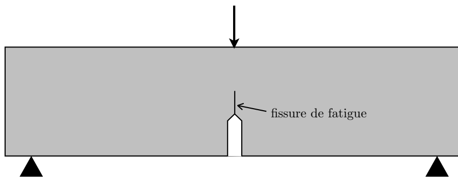
FIGURE 5.15 – Essai de flexion 3 points permettant de mesurer la ténacité K_{Ic} d'un matériau.
