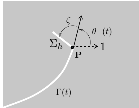
FIGURE 7.11 – Branchement virtuel servant à tester la stabilité de l'état de la structure à l'instant t d'énergie potentielle G(\zeta) associé à ce branchement virtuel dans la direction \zeta est donné par
