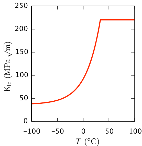
FIGURE 5.16 – Courbe empirique (ici, pour un acier) de dépendance de la ténacité par rapport à la température. La ténacité est pratiquement constante au delà de la température de transition fragile–ductile (ici, environ 30 ^{\circ}\text{C} ). Elle décroît très vite lorsque la température baisse.
