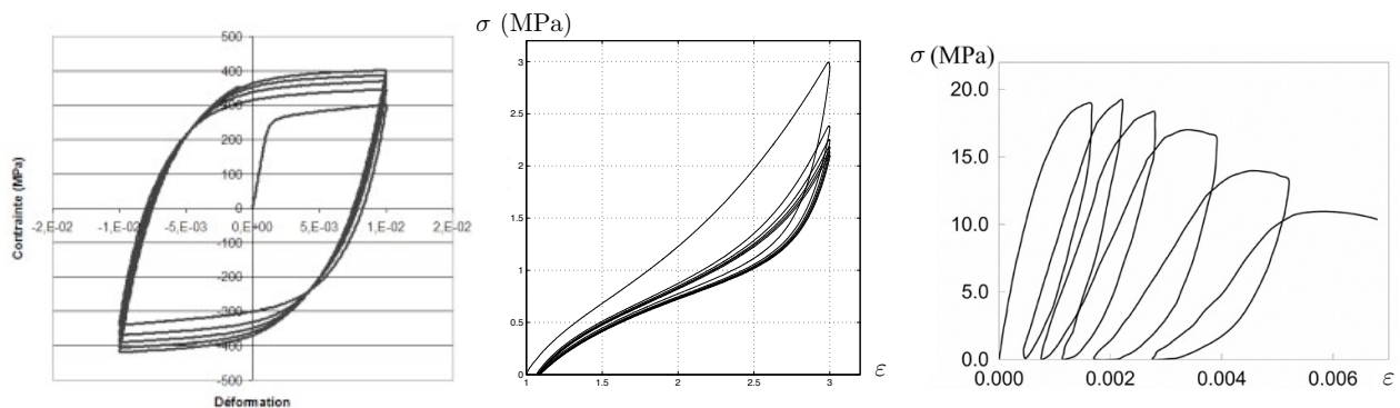
FIGURE 2.5 – Réponses des différents matériaux sous chargement cyclique : à gauche, plasticité cyclique d'un acier ; au milieu, adoucissement cyclique d'un élastomère ; à droite, comportement hystérétique d'un béton en compression
