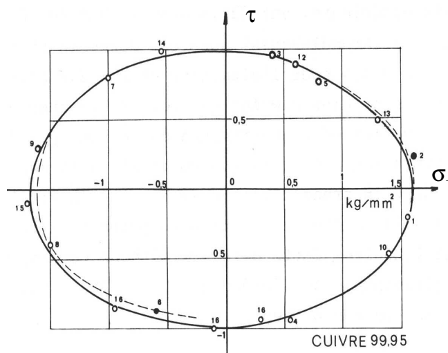
FIGURE 3.25 – Identification du domaine de réversibilité pour du cuivre dans un essai de traction-torsion, Bui (1970).
