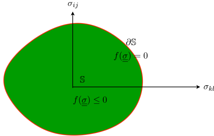
FIGURE 3.11 – Le domaine d'élasticité (en vert) et la surface seuil de plasticité (en rouge) dans l'espace des contraintes.
