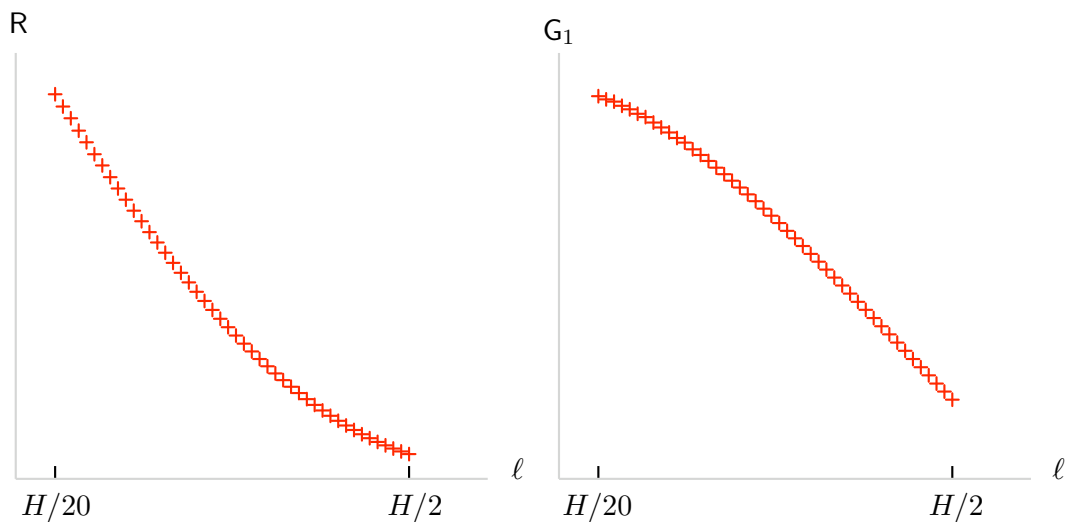
FIGURE 7.5 – Rigidité effective et taux de restitution d'énergie potentielle calculés pour différentes longueurs de fissure dans l'essai de flexion 3 points de la poutre soumise à un déplacement unitaire du point central (l'échelle de valeurs n'a pas d'importance, seules les variations relatives des quantités comptent). On notera la décroissance de G_1 sur la plage de valeurs calculées.
