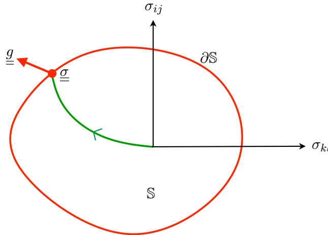
FIGURE 3.12 – Loi d'évolution de la déformation plastique : pas d'évolution de \underline{\underline{\epsilon}}^p tant que \underline{\underline{\sigma}} reste à l'intérieur du domaine de réversibilité actuel et évolution possible de \underline{\underline{\epsilon}}^p dans une direction donnée lorsque \underline{\underline{\sigma}} atteint le seuil de plasticité.
