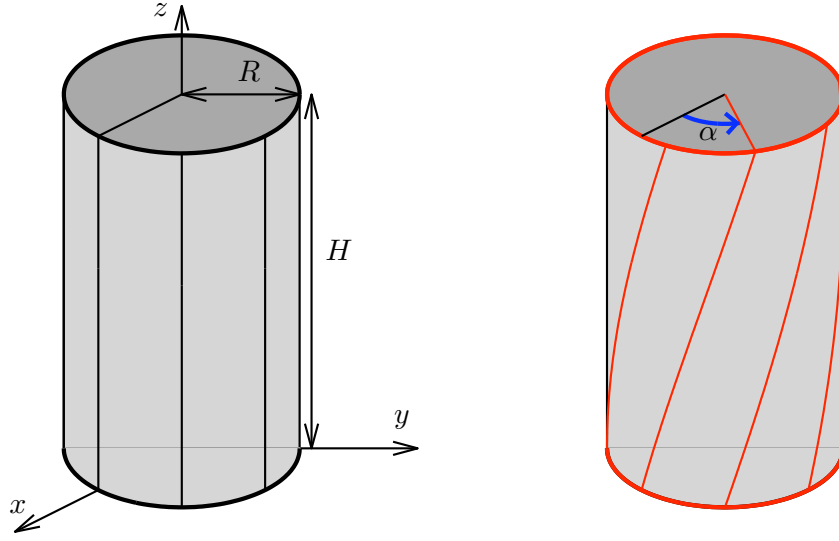
FIGURE 4.1 – Torsion d'un arbre cylindrique à section circulaire. À gauche : configuration de référence ; à droite : configuration déformée.
