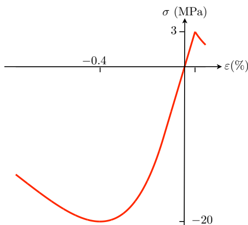
FIGURE 2.3 – Asymétrie du comportement du béton entre la traction et la compression.
