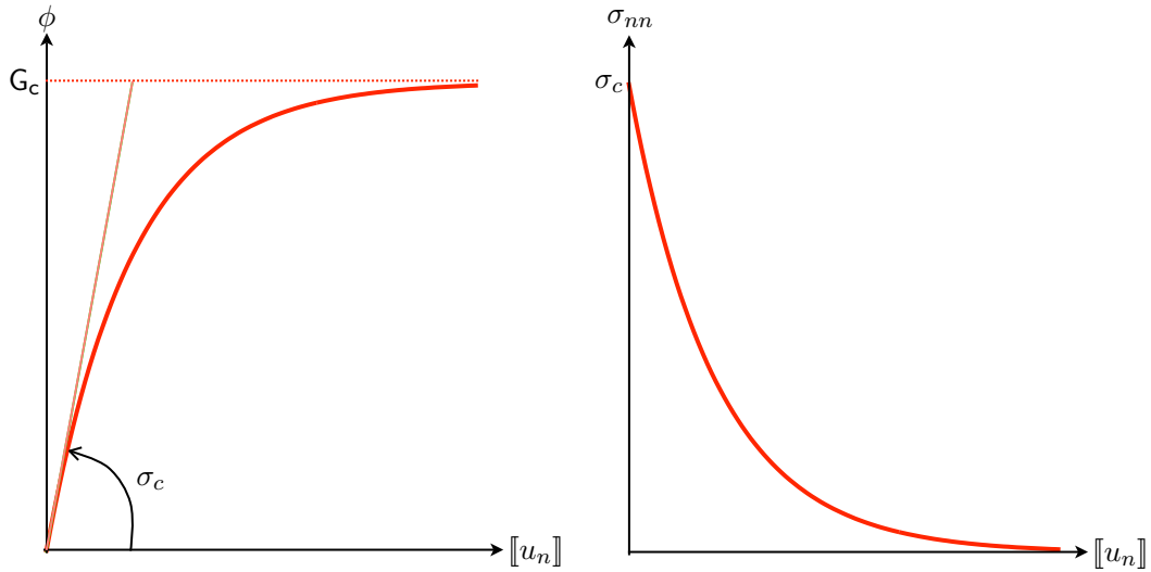
FIGURE 7.14 – Modèle de Barenblatt : la densité d'énergie de fissuration (à gauche) et la contrainte de cohésion (à droite) en fonction du saut de déplacement normal
