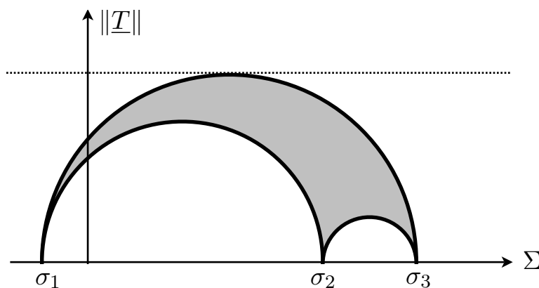
FIGURE 3.22 – Détermination du cisaillement maximal à l'aide des cercles de Mohr.
