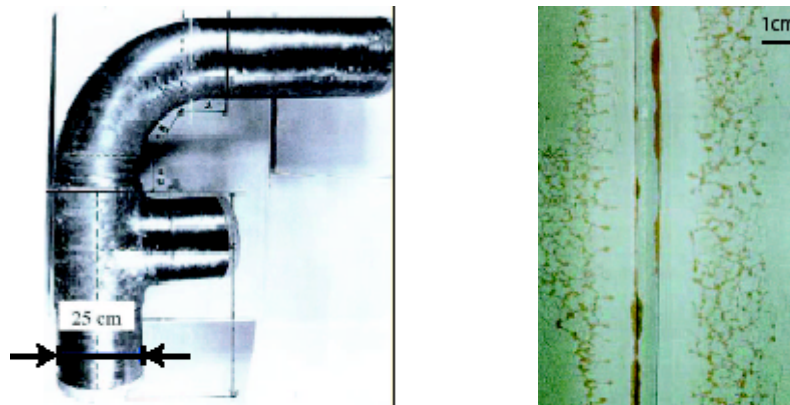
FIGURE 2.14 – Faïençage thermique observé à Civaux dans le tuyau incriminé lors de l'incident du 12 mai 1998.
