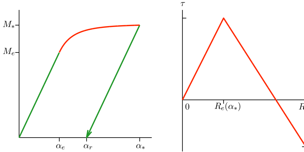
FIGURE 4.6 – À gauche : Réponse globale du cylindre sous chargement de torsion suivi d’une décharge ; à droite, cisaillements résiduels à la fin de la décharge.
