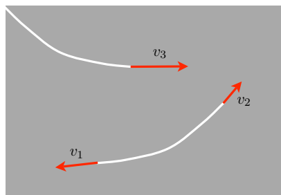
FIGURE 6.1 – Avancée virtuelle des différentes pointes de fissure
