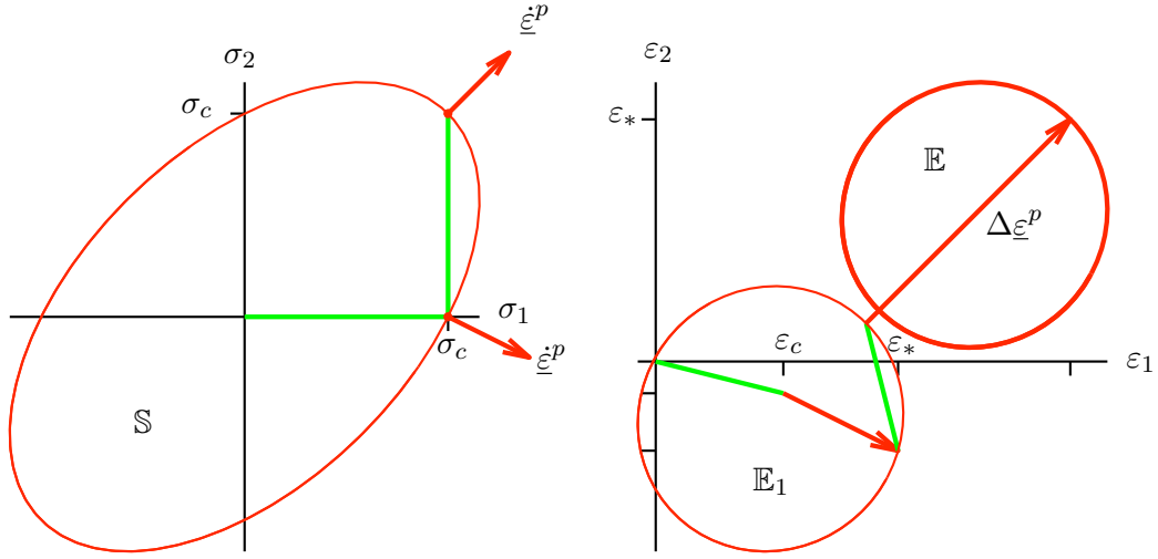
FIGURE 3.20 – La réponse du matériau lors des deux phases de chargement de l’essai-biaxial asymétrique (en vert le trajet correspondant à la phase élastique). À gauche : dans le plan des contraintes ; à droite : dans le plan des déformations.
