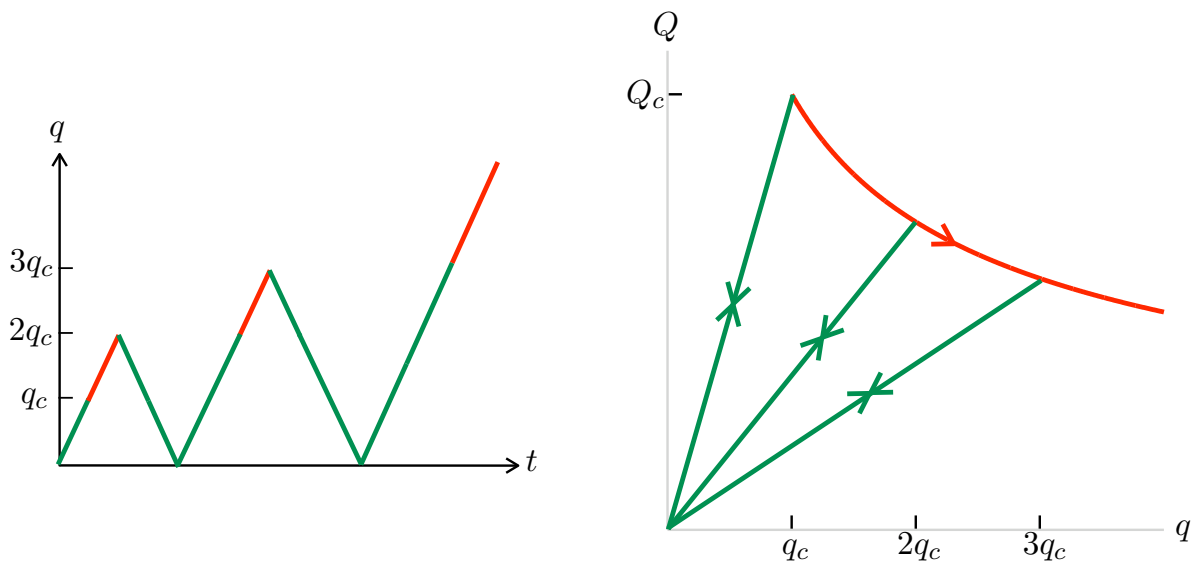
FIGURE 7.2 – Réponse de la poutre DCB sous un déplacement contrôlé non monotone.
