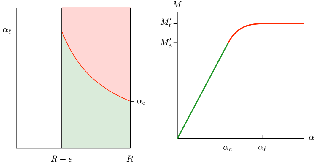
FIGURE 4.3 – Réponse de l'arbre creux sous une torsion croissante. À gauche : pénétration progressive à partir de \alpha_e de la zone plastique vers la surface intérieure qu'elle atteint en \alpha_l ; à droite : réponse globale moment de torsion-angle de torsion, le couple limite M'_l est atteint en \alpha_l .
