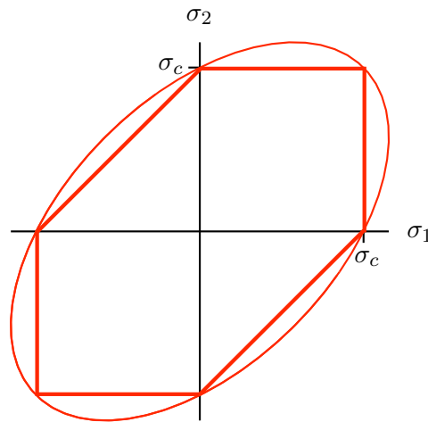
FIGURE 3.23 – L'hexagone de Tresca et l'ellipse de Von Mises dans un essai bi-axial.
