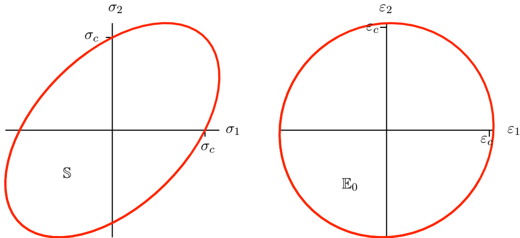
FIGURE 3.18 – L'ellipse de Von Mises dans un essai à contraintes bi-axiales et son image dans le plan des déformations associées en l'absence de déformation plastique (pour \nu = 0.25 ).
