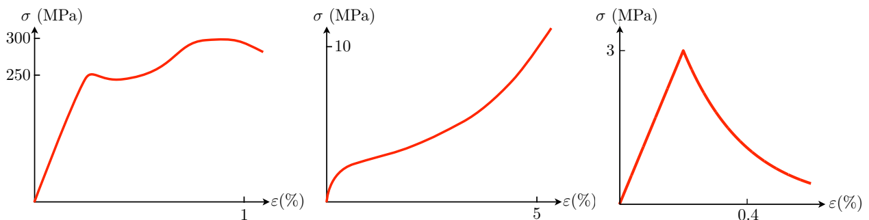
FIGURE 2.2 – Réponses schématiques de différents matériaux dans un essai de traction uniaxiale : à gauche, pour un acier ; au centre, pour un élastomère ; à droite, pour du béton.
