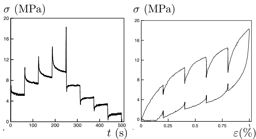
FIGURE 2.8 – Mise en évidence du comportement viscoélastique d'un polymère : à gauche, contrainte uni-axiale \sigma en fonction du temps ; à droite, réponse dans le diagramme (\epsilon, \sigma)
