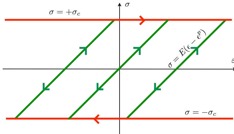
FIGURE 3.4 – Diagramme résumant le comportement de l'assemblage patin-ressort. En rouge : les phases irréversibles de glissement du patin ; en vert : les phases réversibles de blocage du patin.
