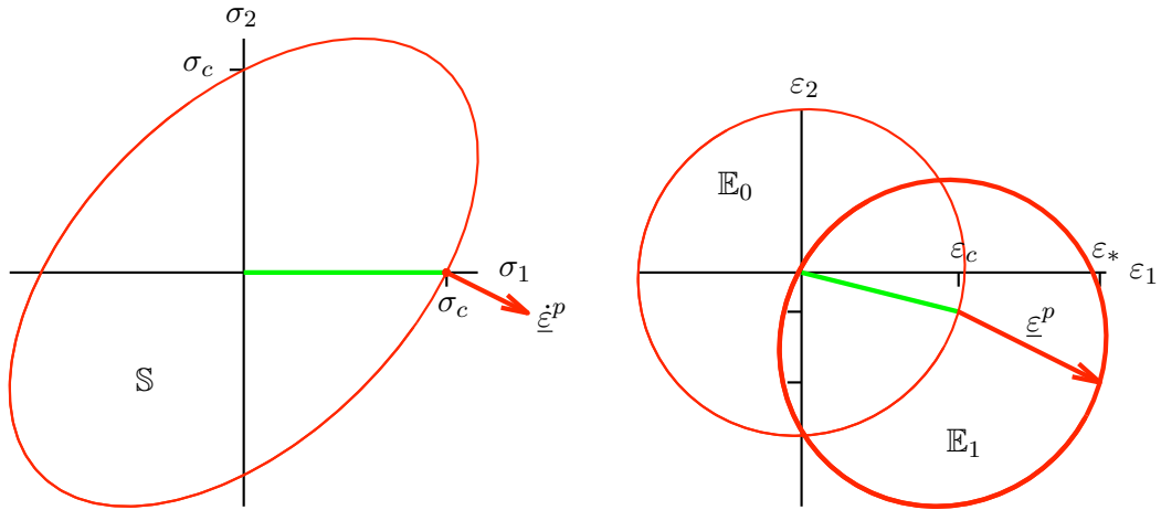
FIGURE 3.19 – La réponse du matériau lors de la première phase de chargement de l’essai-biaxial asymétrique (en vert le trajet correspondant à la phase élastique). À gauche : dans le plan des contraintes ; à droite : dans le plan des déformations.
