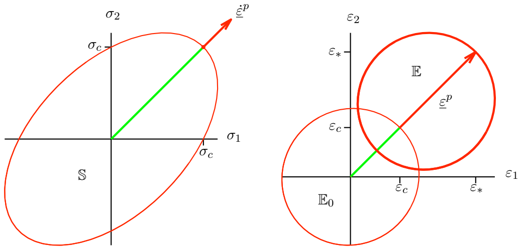
FIGURE 3.21 – La réponse du matériau lors des deux phases de chargement de l'essai-biaxial symétrique (en vert le trajet correspondant à la phase élastique). À gauche : dans le plan des contraintes ; à droite : dans le plan des déformations (pour \nu = 0.25 ).
