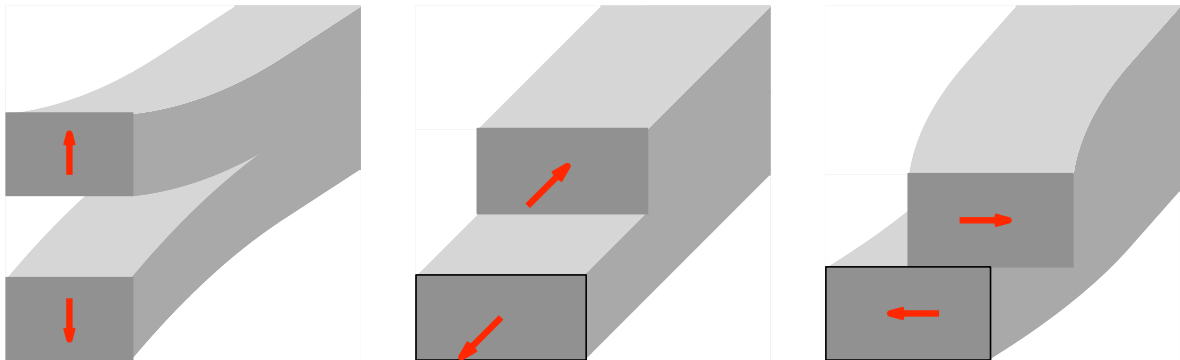
FIGURE 5.12 – Les trois modes singuliers : à gauche, le mode I ou mode d'ouverture ; au centre, le mode II ou mode de glissement ; à droite le mode III ou mode de déchirure.
