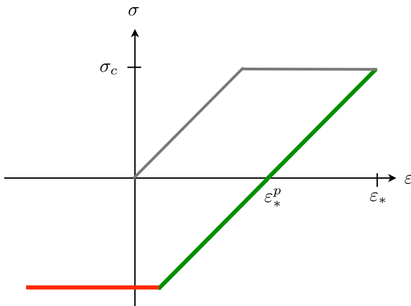
FIGURE 3.3 – Réponse de l’assemblage patin-ressort lors de la décharge. En vert : phase de blocage du patin ; en rouge : phase de glissement du patin vers la gauche.
