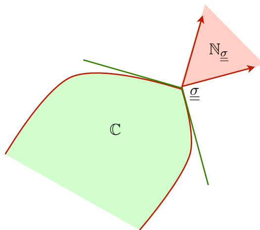
FIGURE 3.16 – Cône (en rouge) des normales extérieures en un point anguleux du bord d'un convexe.
