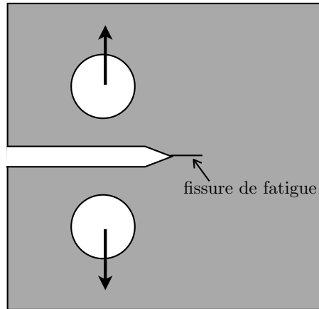
FIGURE 5.14 – Essai sur éprouvette CT permettant de mesurer la ténacité K_{Ic} d'un matériau.
