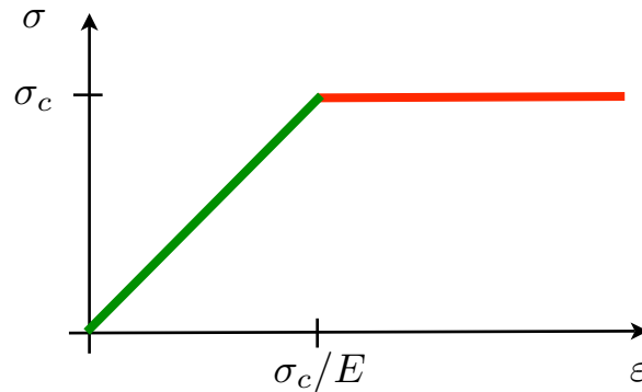
FIGURE 3.2 – Réponse de l'assemblage patin-ressort sous chargement monotone. En vert : phase de mise en tension du ressort ; en rouge : phase de glissement du patin.
