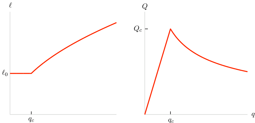
FIGURE 7.1 – Réponse de la poutre DCB sous déplacement contrôlé. À gauche, évolution de la fissure en fonction du déplacement ; à droite, évolution de la force associée en fonction du déplacement. Noter le phénomène d'adoucissement, i.e. la diminution de la force durant la phase d'évolution de la fissure.
