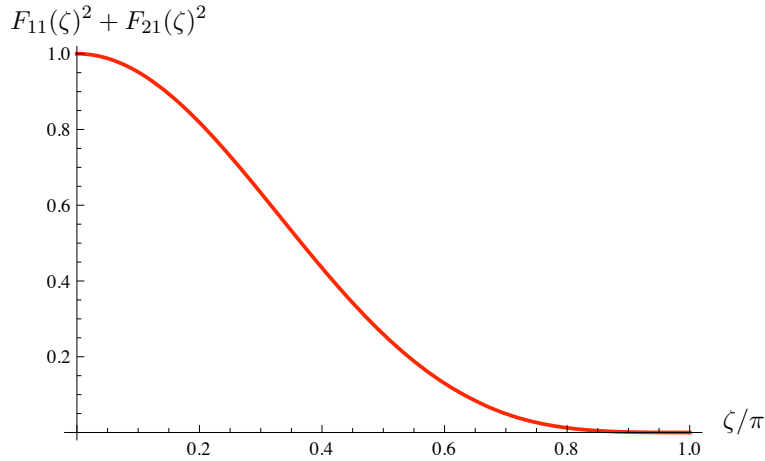
FIGURE 7.12 – Vérification numérique que G(\zeta) est maximal en \zeta = 0 quand K_{II} = 0 .
