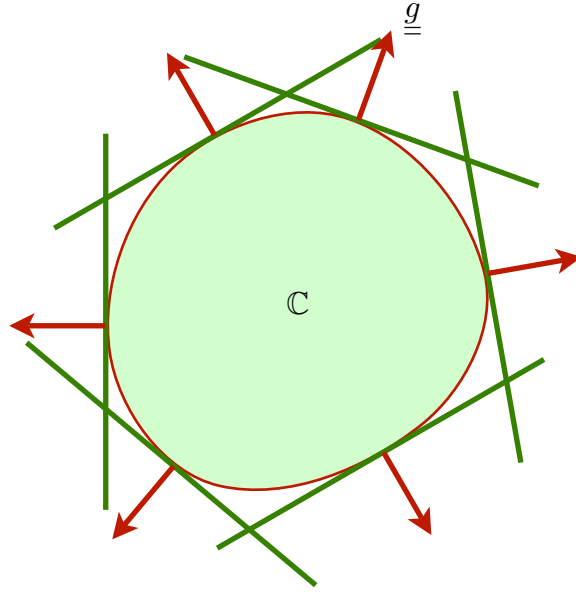
FIGURE 3.17 – Caractérisation d'un convexe par l'intersection des demi-espaces tangents.
