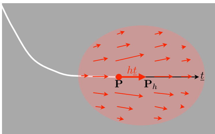
FIGURE 6.4 – Zone de l'objet au voisinage de la pointe de la fissure \mathbf{P} et représentation du champ de vecteur \underline{v} servant à transporter \Omega \setminus \Gamma sur \Omega \setminus \Gamma_h .
