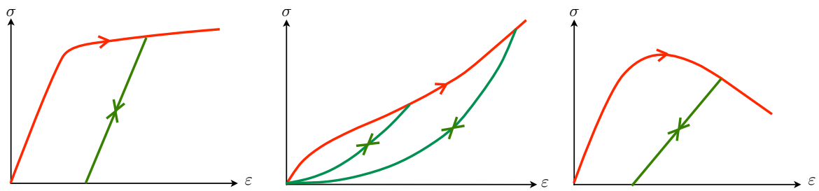
FIGURE 2.4 – Réponses schématiques des différents matériaux dans un cycle de charge-décharge-recharge : à gauche, pour un acier doux ; au centre, pour un élastomère ; à droite, pour un béton en compression.
