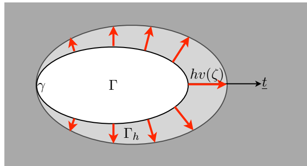
FIGURE 6.2 – Avancée virtuelle du front \gamma de la fissure plane \Gamma
