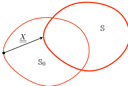
FIGURE 3.13 – Ecrouissage cinématique : translation du domaine de réversibilité.
