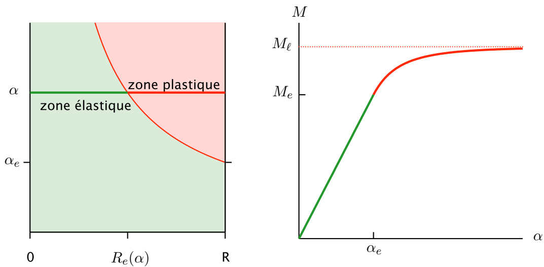
FIGURE 4.2 – Réponse de l'arbre plein sous une torsion croissante. À gauche : pénétration progressive de la zone plastique vers l'axe du cylindre ; à droite : réponse globale moment de torsion-angle de torsion (en vert la phase élastique, en rouge la phase élastoplastique)
