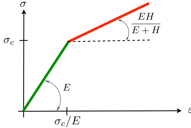
FIGURE 3.7 – Réponse de l’assemblage ressort-patin-ressort sous chargement monotone. En vert : phase de mise en tension du premier ressort ; en rouge : phase de glissement du patin.
