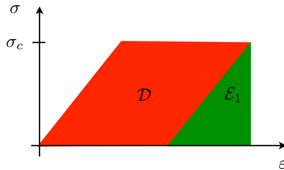
FIGURE 3.5 – Bilan d'énergie de l'assemblage patin-ressort à la fin de la montée en charge. En vert : l'énergie élastique stockée dans le ressort ; en rouge : l'énergie dissipée par frottement.
