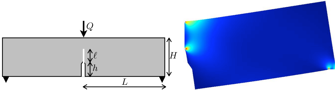
FIGURE 7.4 – À gauche, géométrie de la poutre ; à droite, la déformée de la moitié droite, calculée par la méthode des éléments finis, pour une fissure de longueur H/5 .
