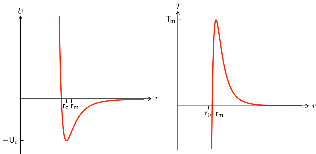
FIGURE 6.5 – Interaction atomique du type Lennard-Jones. À gauche : le potentiel d'interaction ; à droite : la force d'interaction entre deux atomes en fonction de leur distance.
