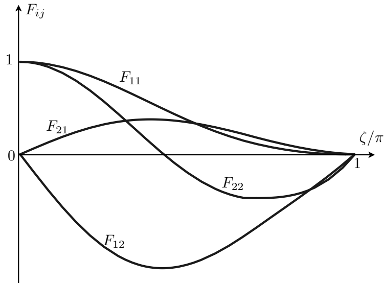
FIGURE 7.10 – Graphe des coefficients F_{ij} donnant les facteurs d'intensité de contraintes après branchement en fonction de l'angle de branchement \zeta .
