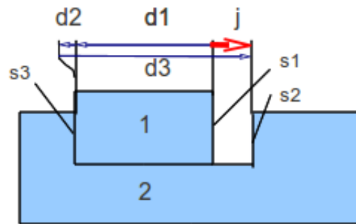
FIGURE 3.32 – Exemple d'une chaîne de cote.
