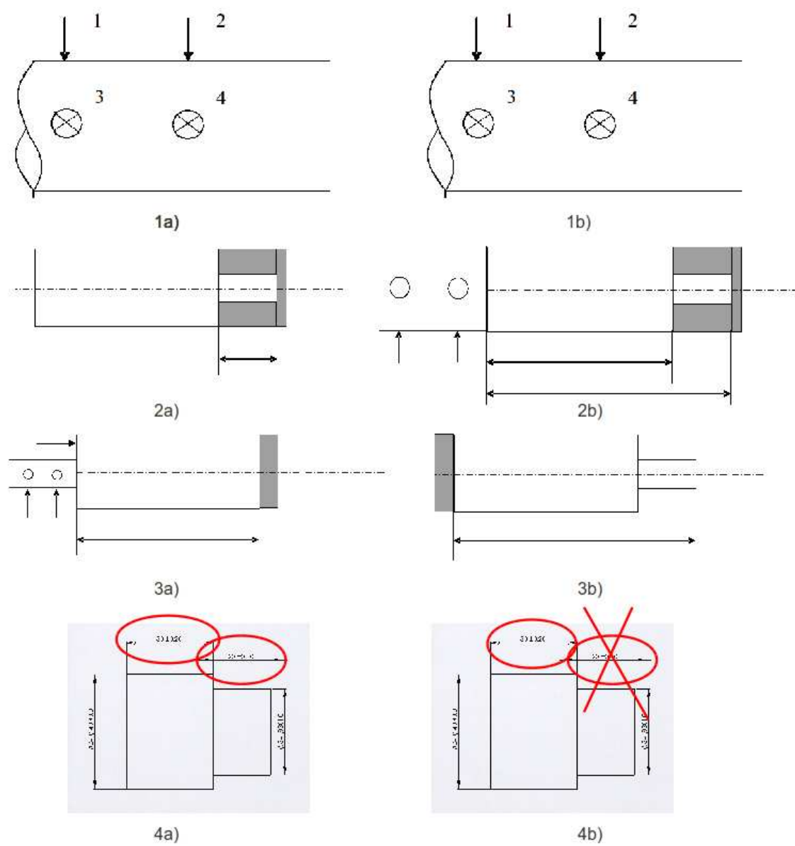
FIGURE 3.38 – Deux procédures d'obtention de la pièce.
