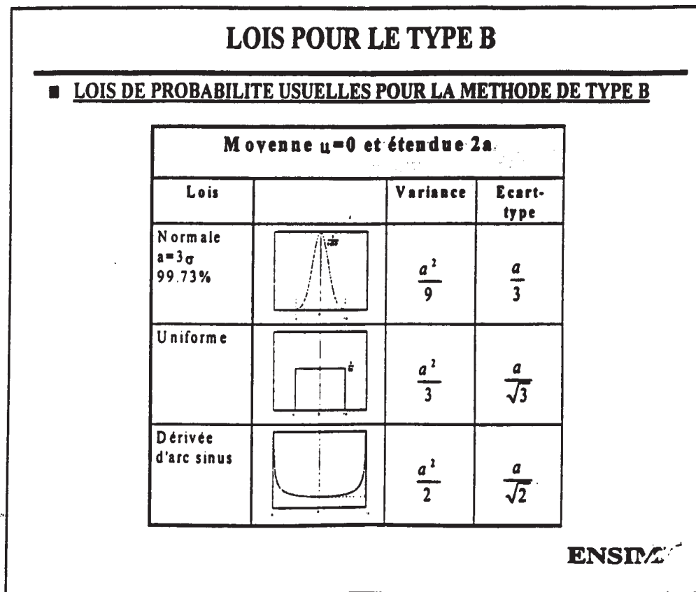
FIGURE 3.21 – Relations entre l'intervalle de tolérance, sa forme et l'écart type.
