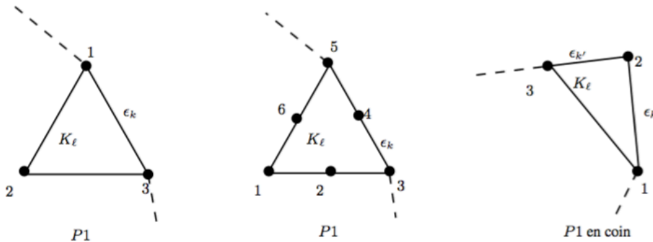
FIGURE 4.7 – Exemples de numérotation d'arête du bord
