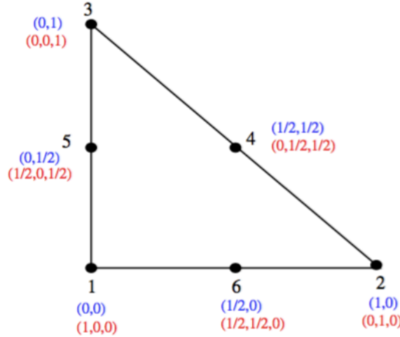
FIGURE 4.6 – Élément de référence pour les éléments finis P2 avec coordonnées cartésiennes et barycentriques des nœuds
