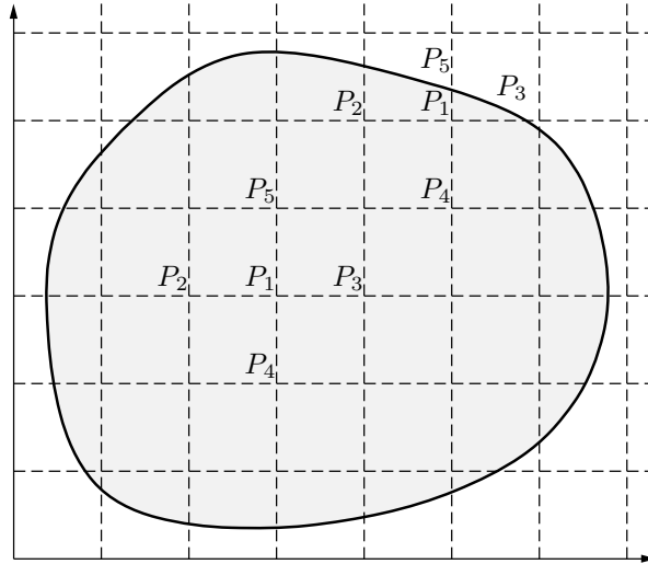
FIGURE 1.4 – Discretisation différences finies bi-dimensionnelle
