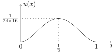
FIGURE 3.6 – Allure de la fonction x \mapsto \frac{1}{24}x^2(1-x)^2
