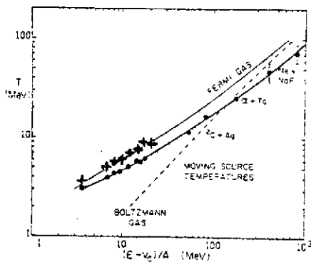
Figure 86 : Température de la boule de feu en fonction de l'énergie incidente corrigée pour la répulsion coulombienne. Les points sont expérimentaux pour les protons (points noirs) et les deutérons (croix).
