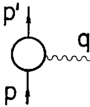
Fig.8 - Couplage électromagnétique photon-nucléon dans le milieu.
