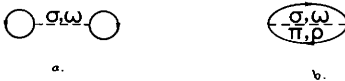
Fig.3 - Contribution du terme direct (a. Hartree) et d'échange (b. Fock) à l'énergie
