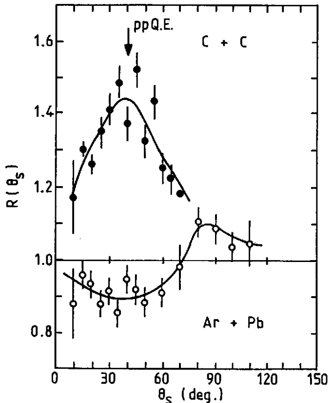
Fig.23 Même dispositif expérimental que celui décrit dans la figure 22a. Variation du rapport de coïncidence dans et hors plan en fonction de l'angle du spectromètre. Les lignes --- ne sont là que pour guider l'oeil. Data réf. 75 .
