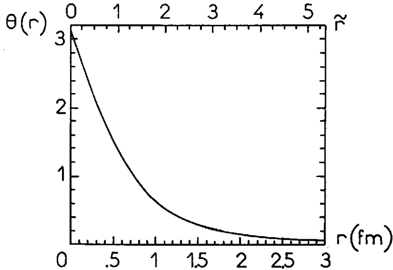
Fig 1 : Solution de l'équation (21) satisfaisant aux conditions (22) avec n = 1 , e = 545 , f_\pi = 64,5 et \tilde{r} = e f_\pi r (ref. 11).
