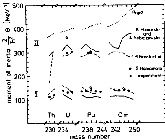
Fig.13. Moments d'inertie des actinides dans l'état isomérique et l'état fondamental, comparés à différents résultats de calculs.
