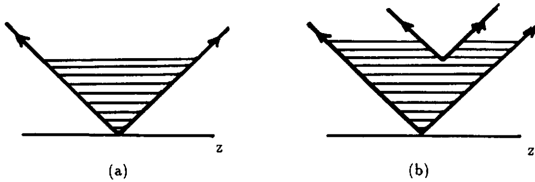
Figure 25: Représentation d'un tube de flux dans le diagramme (t,z) , dans le référentiel du centre de masse de la paire quark-antiquark; (a) état initial, (b) configuration après brisure du tube de flux en un point.
