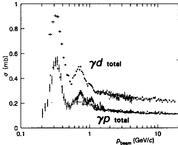
Figure 10 Section efficace totale d'absorption de photons sur le proton et le deuteron 2) .
