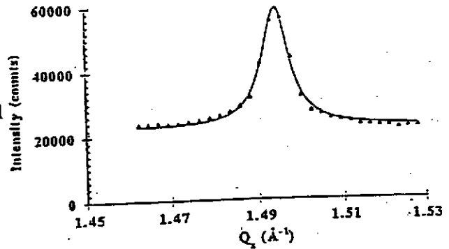
Fig. 8 a) Diffractogramme de poudre d'une monocouche de 1-dodécanol à 10,5°C en fonction du moment parallèle Q_x
