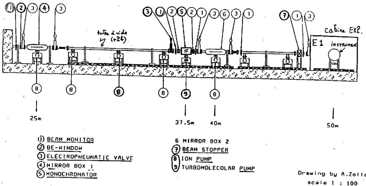
Fig. 1 Ligne de rayons X générique : seule la partie dans le hall expérimental est schématisée (partie située entre 25 m et ≈50-70 m de la source synchrotron); à noter que les composants optiques principaux (monochromateur, miroir) sont souvent placés dans une cabine plombées, tout comme les instruments.
