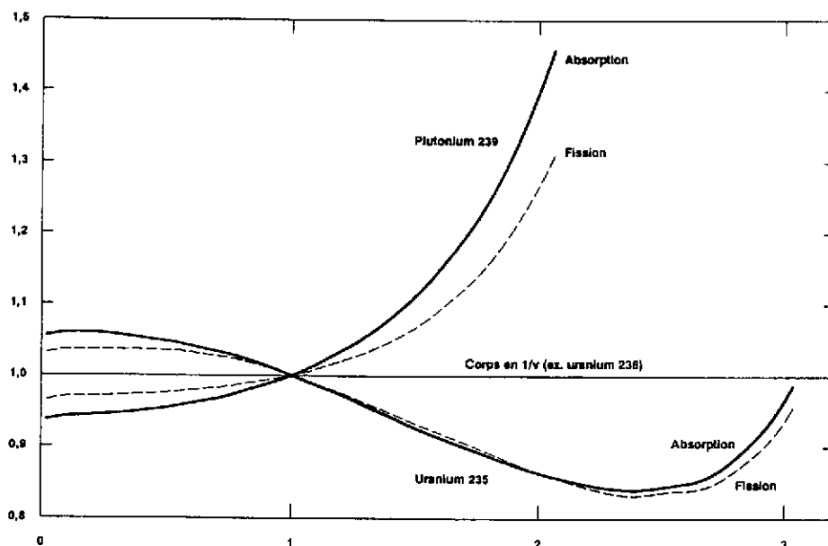
Produit vitesse * section efficace (rapporté à sa valeur à 2 200 m/s) en fonction de la vitesse (rapportée à 2 200 m/s)
