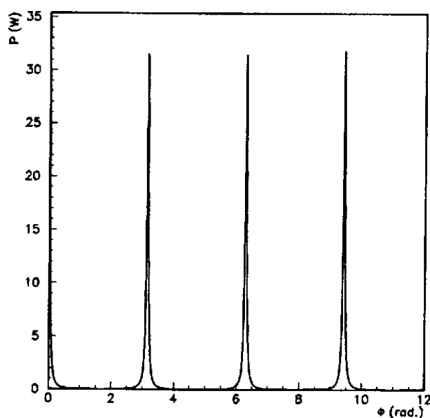
Figure 18: Fonction d'Airy représentant la puissance dans une cavité en fonction de l'accord de phase \phi .
