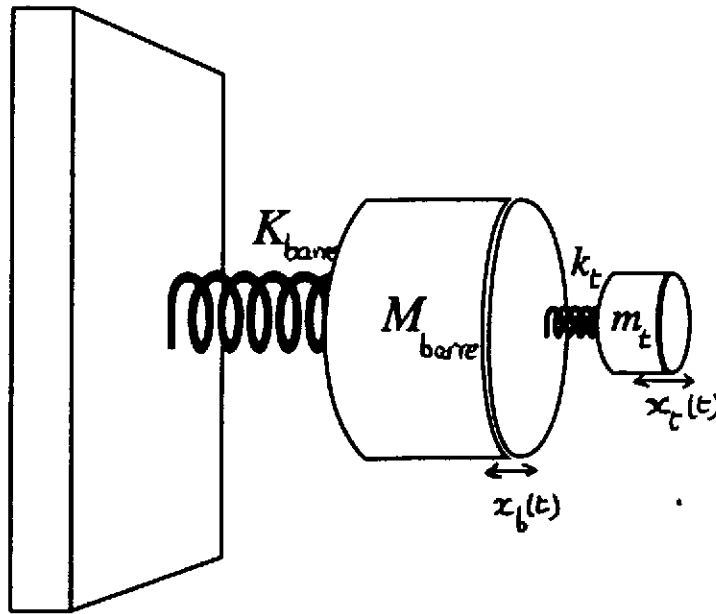
Figure 5: Schéma mécanique du système barre+transducteur
