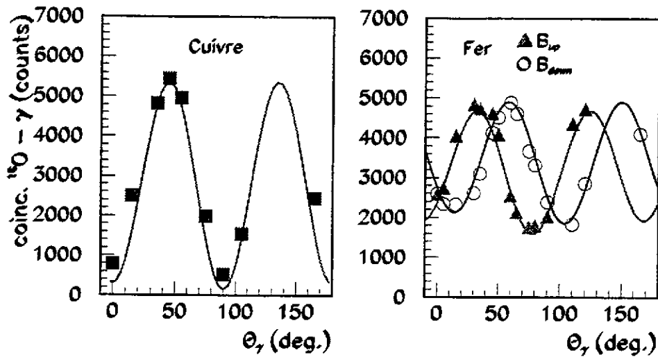
figure 7 : distributions angulaires du rayonnement \gamma en coïncidence avec des projectiles retrodiffusés pour la réaction ^{148}\text{Nd}(^{16}\text{O}, ^{16}\text{O} \ 7300\text{keV})^{140}\text{Nd} à E_{^{16}\text{O}} = 35\text{ MeV} . Les données expérimentales sont de Ben Zvi et al. [5]. Gauche : avec un support de cuivre. La courbe est la distribution angulaire théorique sans effet de déorientation. Droite : avec un support de fer et deux orientations d'un champ magnétique appliqué. Les courbes sont des ajustements tenant compte d'un décalage angulaire et d'un amortissement de l'amplitude d'oscillation dus à l'effet de déorientation.
