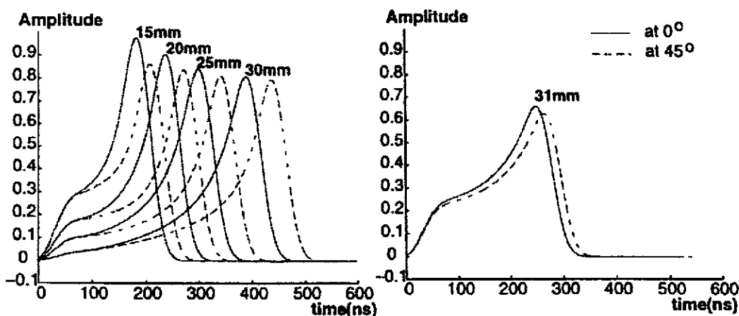
Figure 17 : Impulsions en courant mesurées dans les parties frontale (gauche) et coaxiale (droite) d'un cristal tronçonné. En traits pleins les impulsions correspondant à une collection selon l'axe \langle 100 \rangle et en pointillés celles selon l'axe \langle 110 \rangle . Les impulsions pour différents rayons d'interaction sont montrées.
