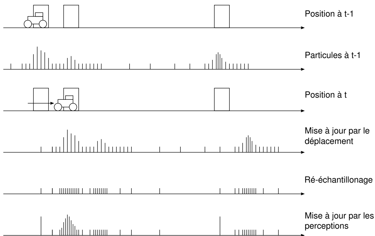
FIGURE 10.19 – Illustration du fonctionnement de l'algorithme de filtrage particulaire. Les particules se concentrent autour des positions de plus forte probabilité.
