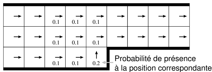
FIGURE 12.7 – Exemple de l'intérêt d'une procédure de vote dans le cas où la situation du robot est incertaine. Si l'on choisit l'action associée à la position la plus probable, le robot ira en haut, ce qui correspondra à l'action correcte avec une probabilité 0,2. En utilisant une méthode de vote, l'action choisie sera d'aller à droite, ce qui sera correct avec une probabilité 0,8.
