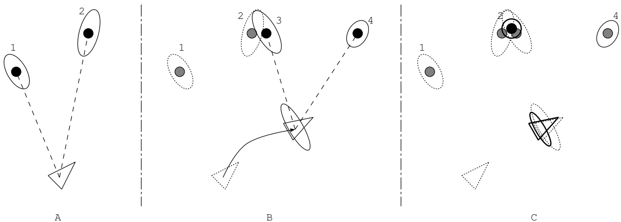
FIGURE 11.10 – Illustration de l'algorithme de SLAM par filtrage de Kalman. Dans la partie A, le robot, dans sa position initiale, perçoit les amers 1 et 2 qui sont ajoutés à la carte. Dans la partie B, le robot s'est déplacé (on dispose d'une estimation bruitée de sa position par l'odométrie) et il perçoit les deux amers 3 et 4. Dans la partie C, on a considéré que les amers 2 et 3 étaient le même amer, ce qui a permis de mieux estimer sa position et de corriger l'estimation de la position du robot. L'amer 4 a été ajouté à la carte.
