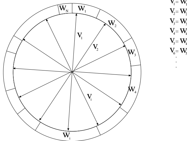
FIGURE 10.17 – Illustration de la méthode d'échantillonnage. L'ensemble de particules w est ré-échantillonné en l'ensemble v .
