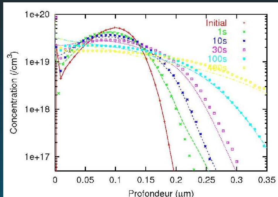
Example of Boron diffusion profile diffusion
