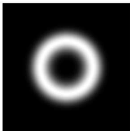
LG(0,1) : vortex
