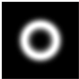
LG(0,1) : vortex
