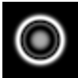
LG(1,3)
