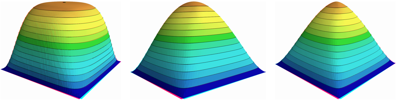
FIGURE 2.4 – Fluide quasi-newtonien à loi de puissance ( n = 0.5, 1, 1.5 ) : écoulement de Poiseuille dans un tuyau de section carré représenté en élévation (d'après [Sar11, part 3]).
