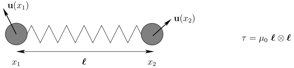
FIGURE 4.1 – Fluides viscoélastiques : une suspension de ressorts élastiques.
