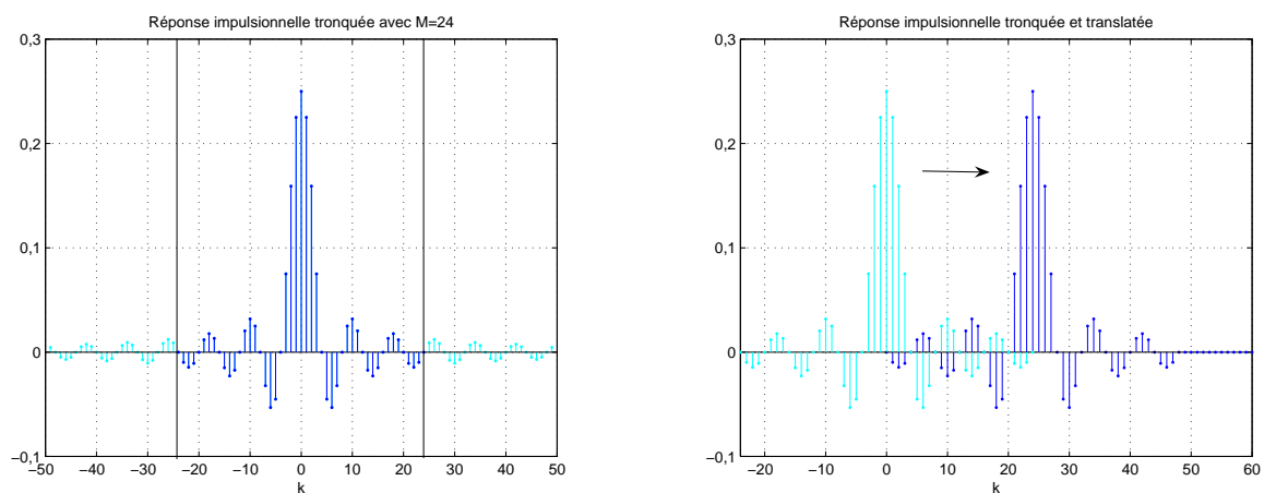
FIG. 6.12 – Réponse impulsionnelle tronquée (gauche) puis translaturée (droite)
