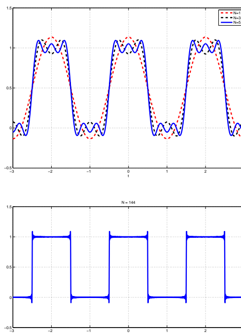
FIG. 2.9 – Somme des N premiers termes de la décomposition en série de Fourier avec N = 1 , N = 3 et N = 5 (haut) et N = 144 (bas)
