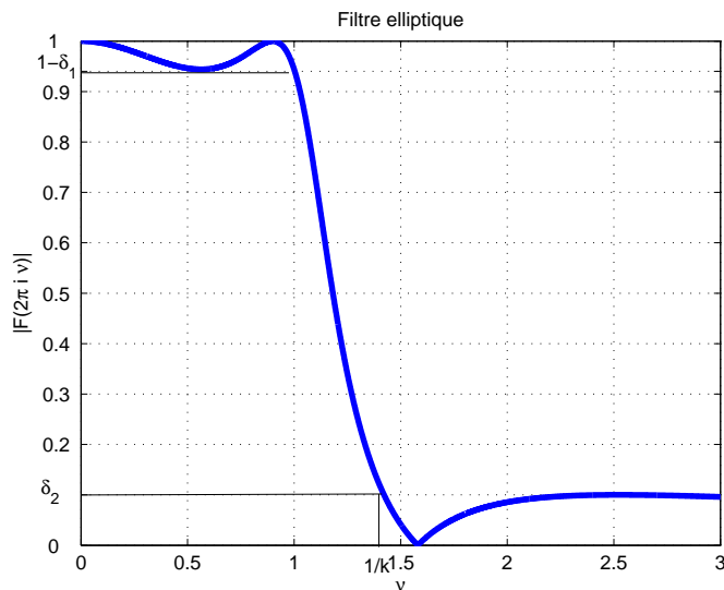
FIG. 3.24 – Filtre elliptique
