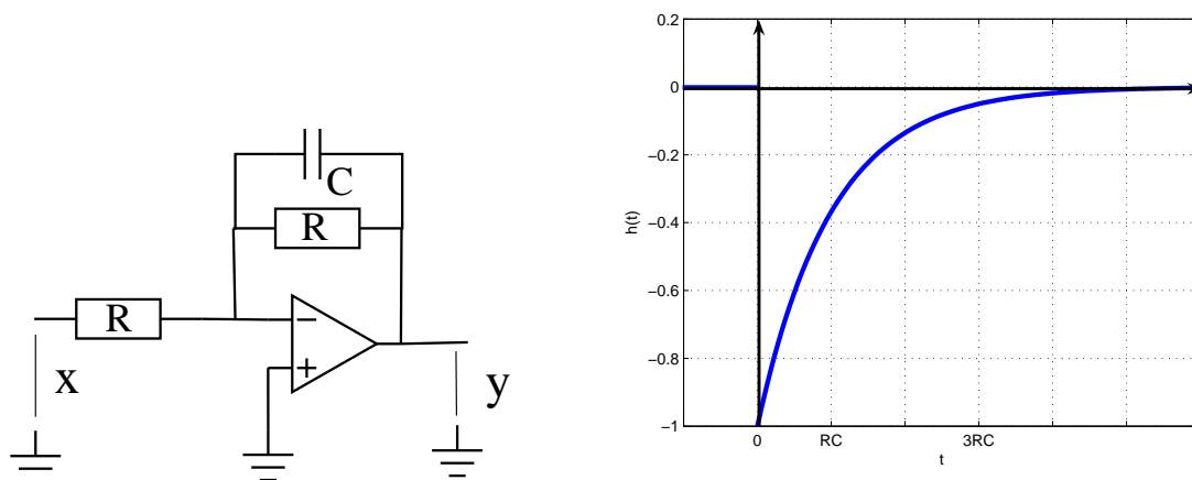
FIG. 3.4 – Exemple de système de convolution
