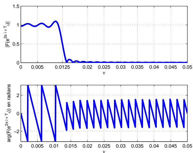
FIG. 6.13 – Réponse fréquentielle du filtre passe-bas RIF
