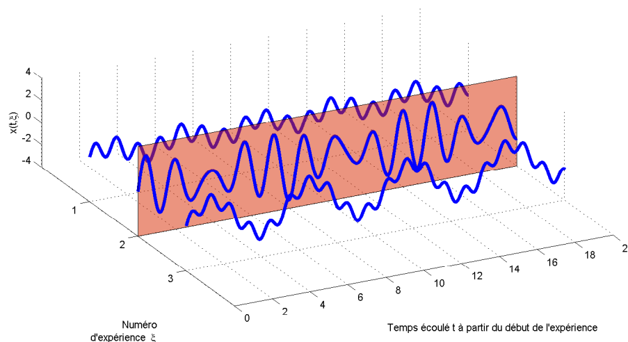
FIG. 7.3 – Notion d'ergodicité
