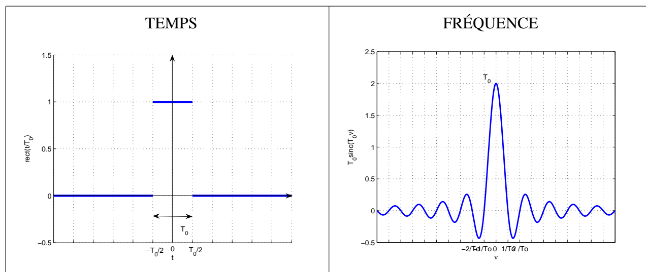
FIGURE 2.12 – Fonction rectangle et sa transformée de Fourier
