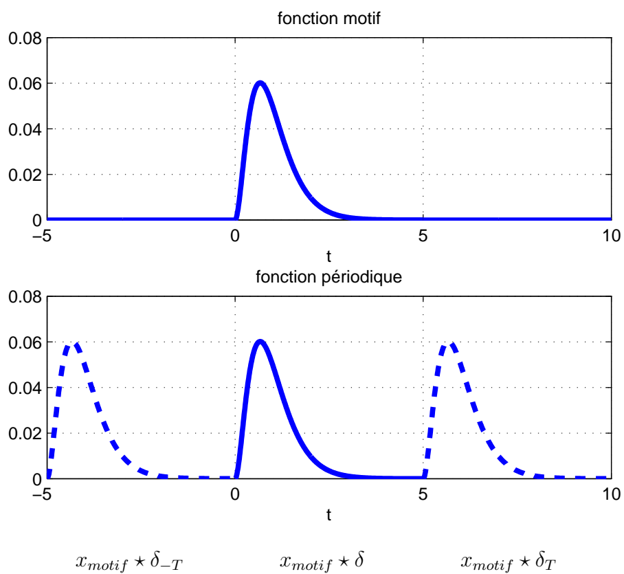
FIGURE 5.21 – Fonction périodique et fonction motif : x = x_{motif} * Pgn_T
