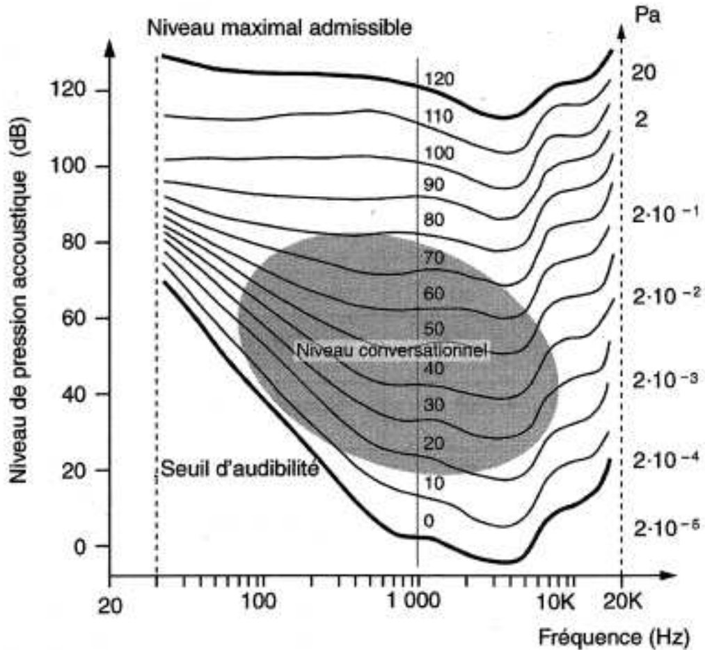
FIGURE 2.25 – Courbes d'audition isononiques : Pression acoustique en Pascal (ordonnée à droite) versus fréquence (abscisse) (extrait de [12])
