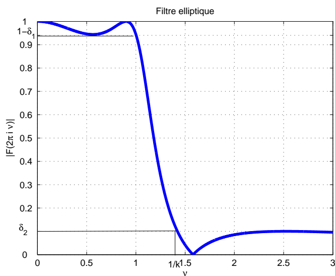
FIGURE 3.29 – Filtre elliptique
