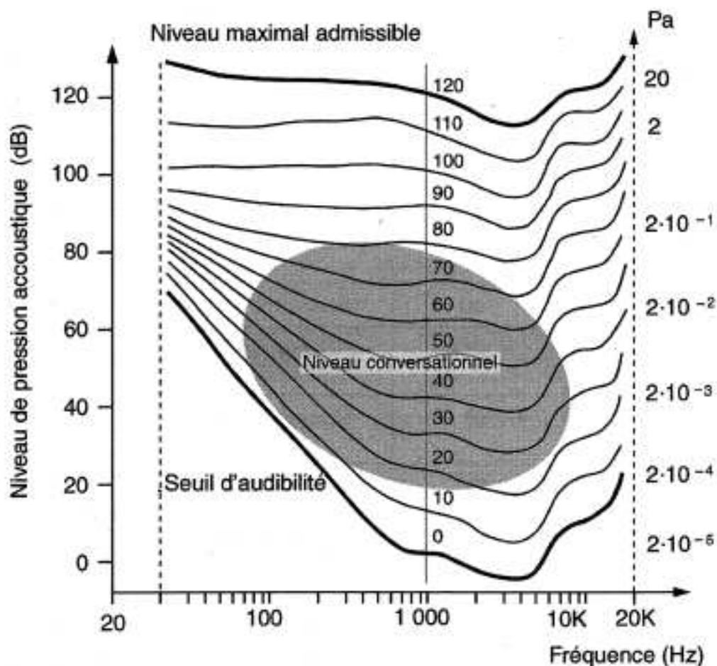
FIGURE 2.25 – Courbes d'audition isoniques : Pression acoustique en Pascal (ordonnée à droite) versus fréquence (abscisse) (extrait de [15])
