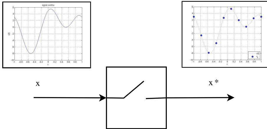
FIGURE 5.2 – Signal échantillonné
