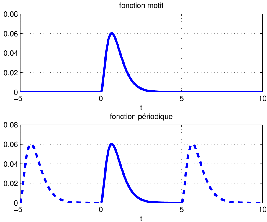
FIGURE 2.25 – Fonction périodique et fonction motif
