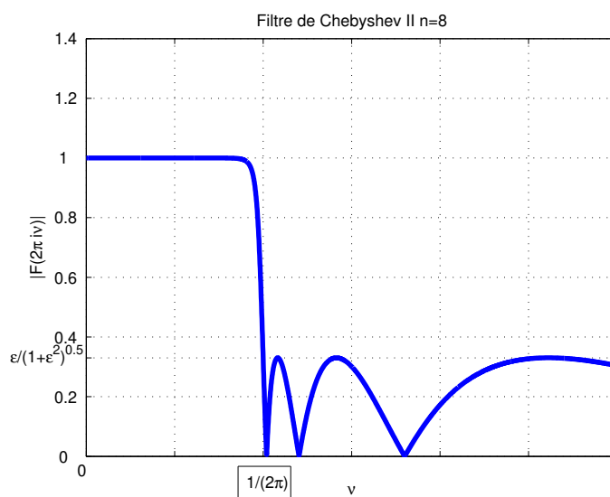
FIGURE 3.28 – Filtrés de Chebyshev de type II
