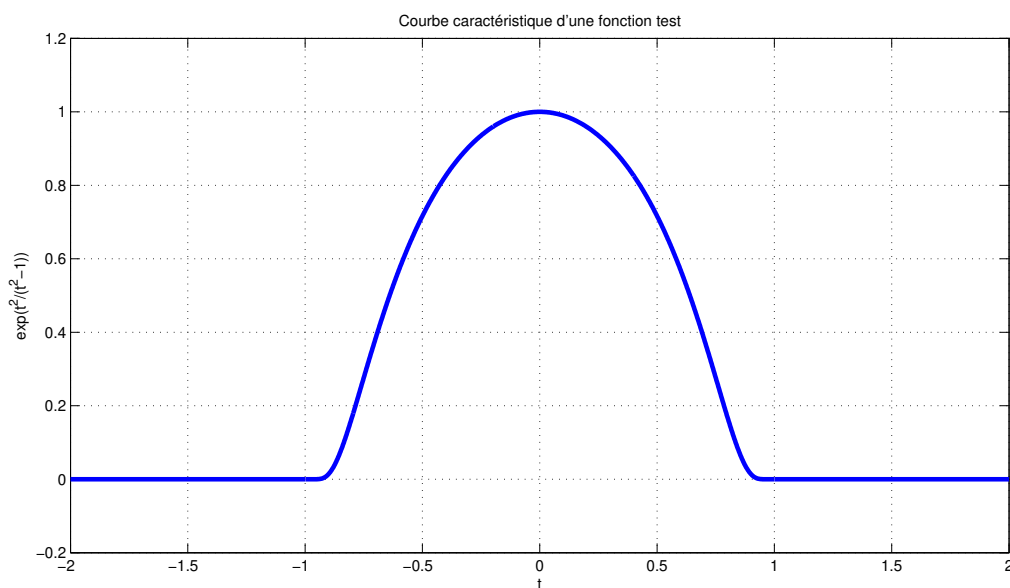
FIGURE 2.21 – Courbe caractéristique d'une fonction test
