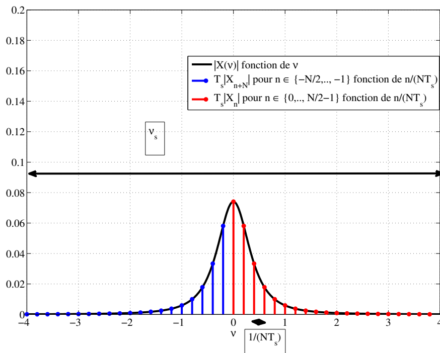
FIGURE 5.25 – Spectre en module |X(\nu)| du signal continu et points obtenus à partir de la TFD
