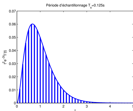
FIGURE 5.20 – Signal x(t) = t^2 e^{-3t} \Gamma(t) (trait continu) et échantillons x_k
