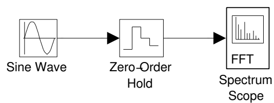
FIGURE 5.28 – Analyseur de Spectre sous Simulink
