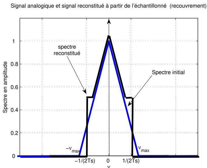
FIGURE 5.10 – Spectre du signal analogique de départ et spectre du signal analogique reconstitué en cas de repliement de spectre
