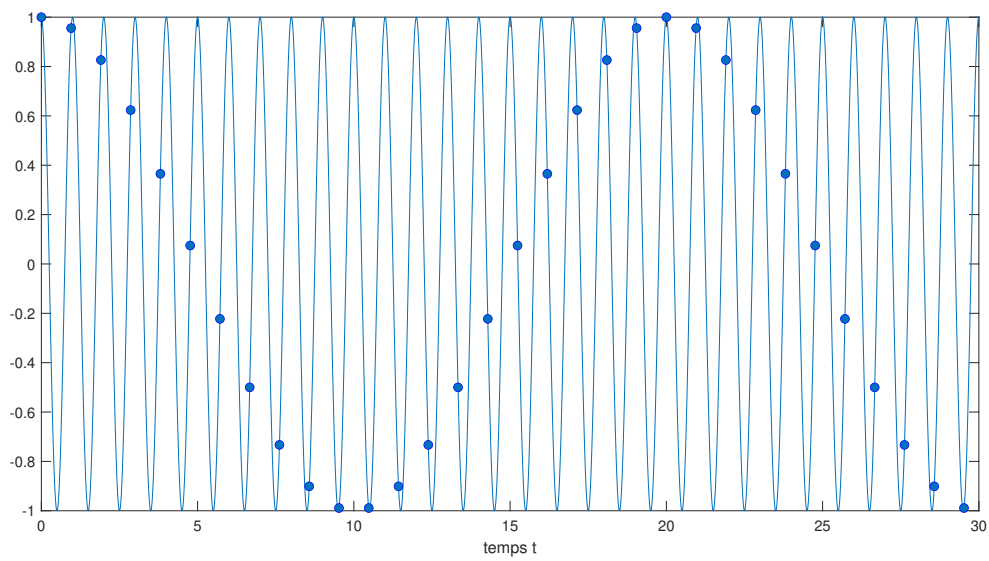
FIGURE 5.13 – Signal analogique x (trait continu) et signal échantillonné (points) à \nu_s = 1.05 Hz
