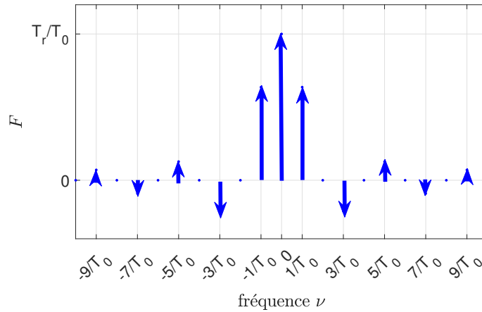
FIGURE 2.24 – Spectre de la fonction périodique de période T_0 associée à la fonction motif \text{rect}\left(\frac{\bullet}{T_r}\right)
