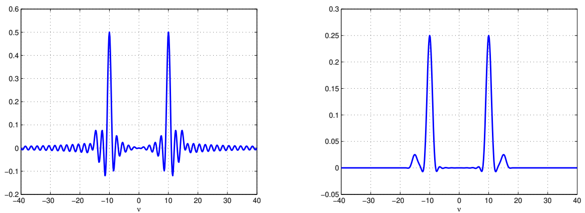
FIGURE 2.36 – Spectre de x_{T_a} (gauche) et de w_{hanning}(t)x_{T_a} (droite)
