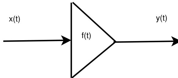
FIGURE 2.30 – Fenêtrage temporel
