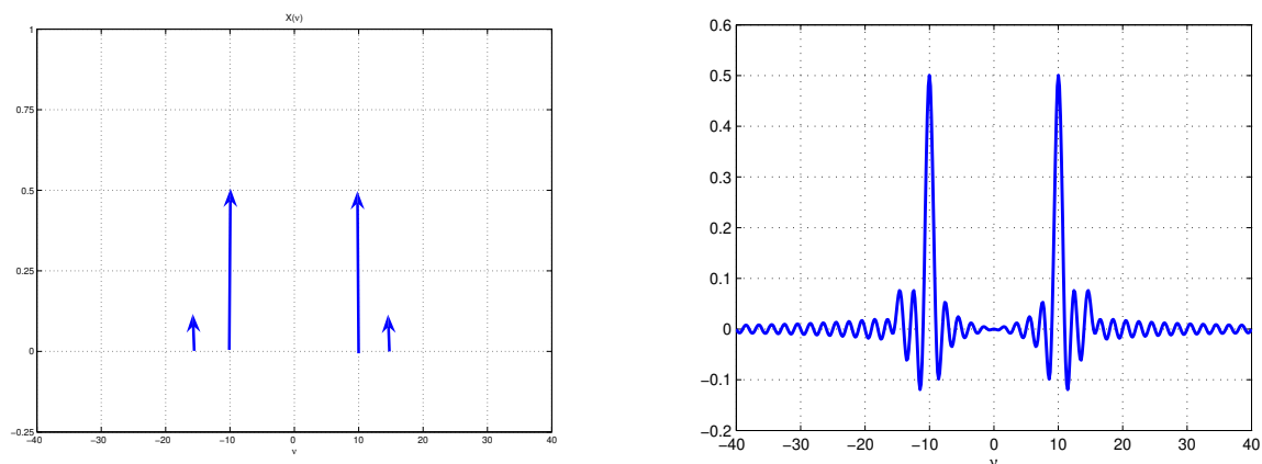
FIGURE 2.29 – Spectre de x (gauche) et de x_{T_a} (droite)
