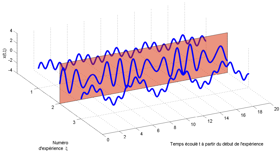
FIGURE 7.7 – Notion d'ergodicité
