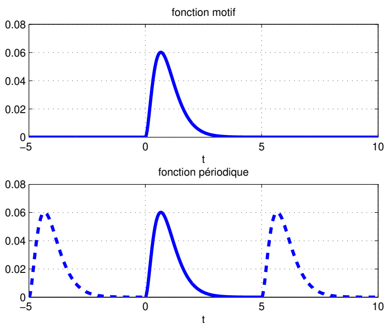
FIGURE 2.25 – Fonction périodique et fonction motif
