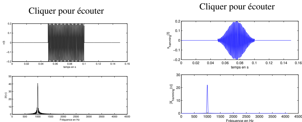
FIGURE 2.39 – Signal sinusoïdal fenêtré
