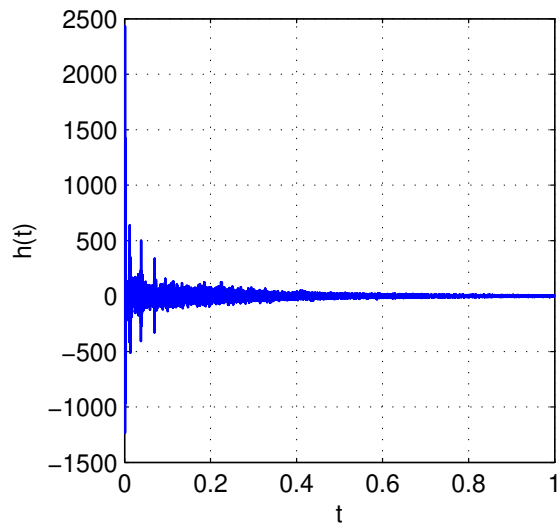
FIGURE 3.11 – Réponse impulsionnelle d'une salle d'église
