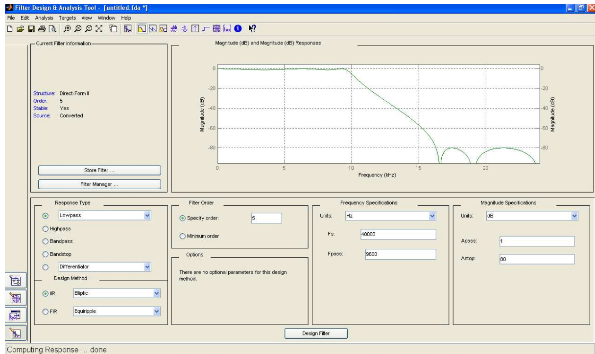
FIGURE 6.26 – Interface graphique fdatool de Matlab
