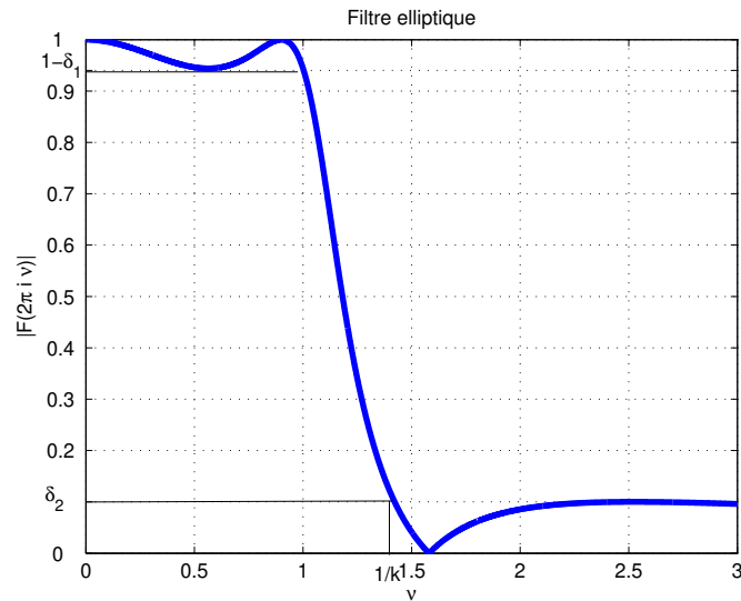
FIGURE 3.30 – Filtre elliptique
