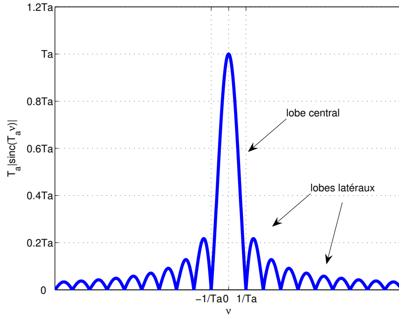
FIGURE 2.31 – Spectre en module d'une fenêtre rectangulaire
