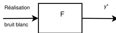
FIGURE 7.13 – Notion de filtre générateur dans le cas d'un signal aléatoire
