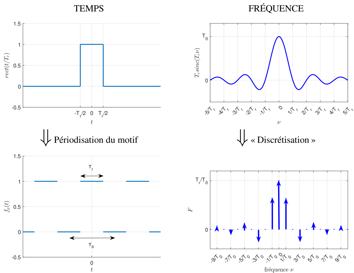
FIGURE 2.26 – Spectre d’une fonction périodique et spectre de la fonction motif correspondante
