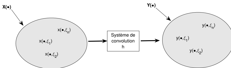
FIGURE 7.10 – Sortie d'un système de convolution pour des entrées réalisations d'un processus aléatoire
