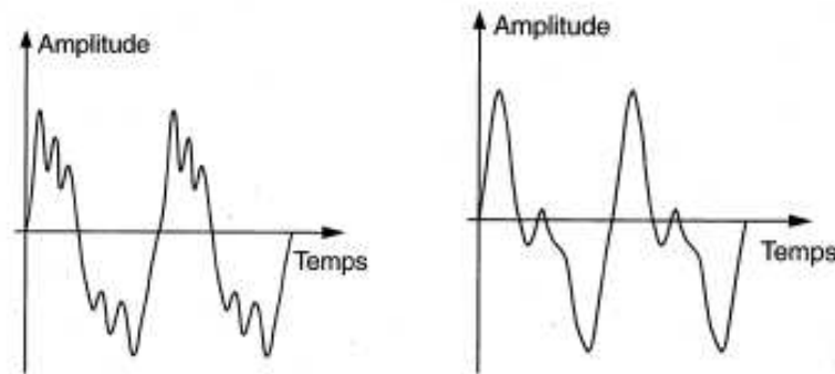
FIGURE 2.37 – Signaux périodiques correspondant à un piano (gauche) et à une clarinette (droite) (extrait de [15])
