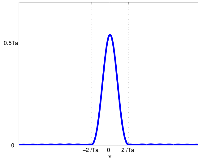
FIGURE 2.34 – Spectre en module de la fenêtre de Hamming
