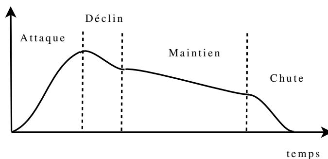
FIGURE 2.38 – Fenêtre temporelle d'instrument de musique
