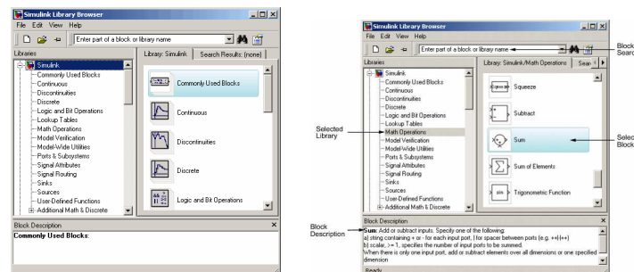
FIGURE 3.34 – Fenêtre Simulink
