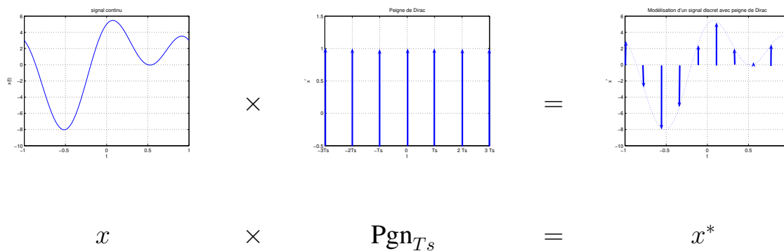
FIGURE 5.6 – Modélisation de l'échantillonnage par peigne de Dirac
