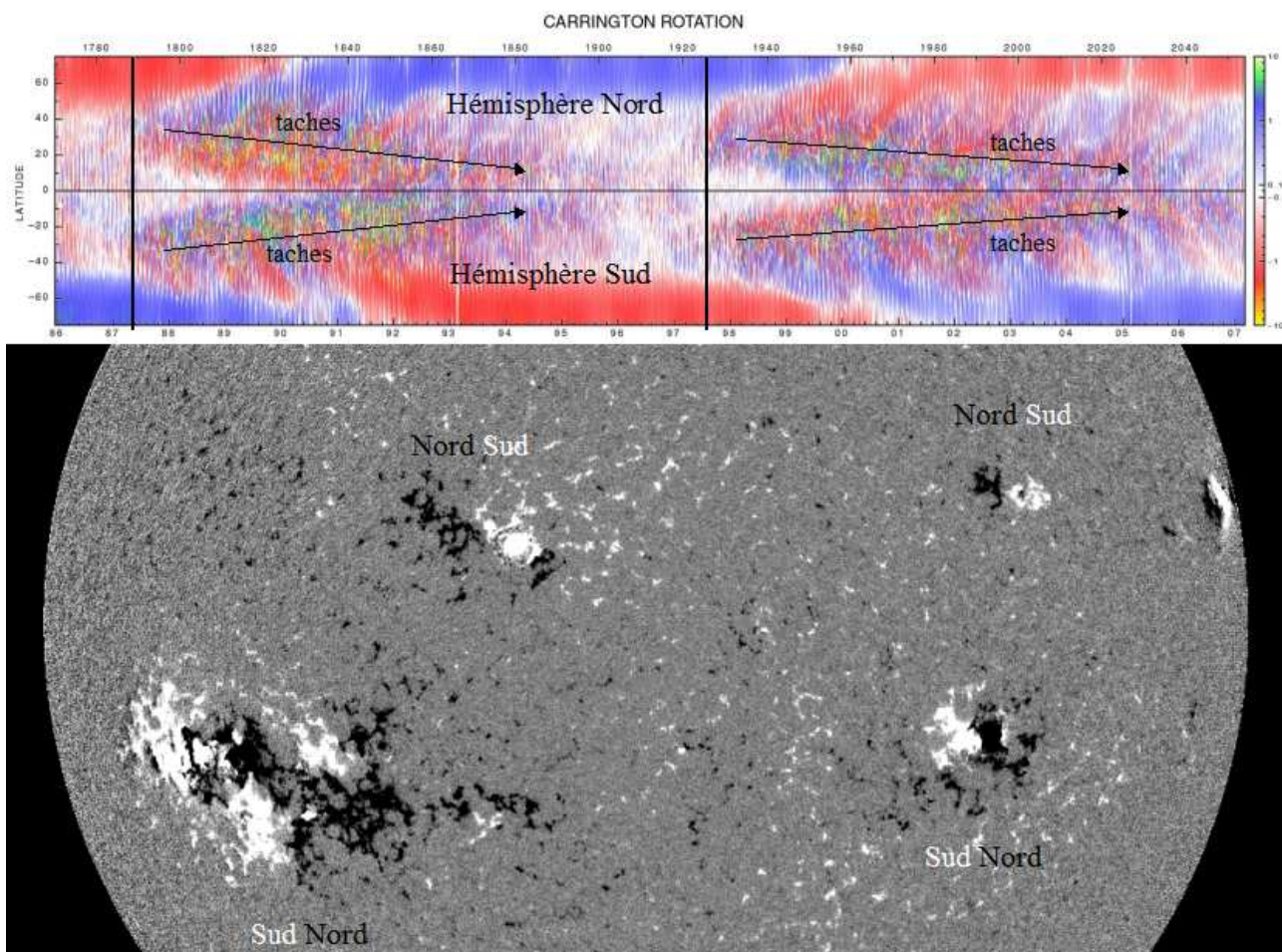
Figure 40 : Cycle magnétique solaire de 22 ans : en haut carte synoptique du Mont Wilson de 1986 à 2007 montrant la distribution des polarités magnétiques Nord et Sud (rouge et bleu) en fonction du temps (croissant de gauche à droite) et de la latitude. Le champ magnétique s'inverse tous les 11 ans. En bas, magnétogramme de SOHO/MDI montrant la différence de polarités entre les taches des régions actives des deux hémisphères (en noir et blanc polarités Nord et Sud).
