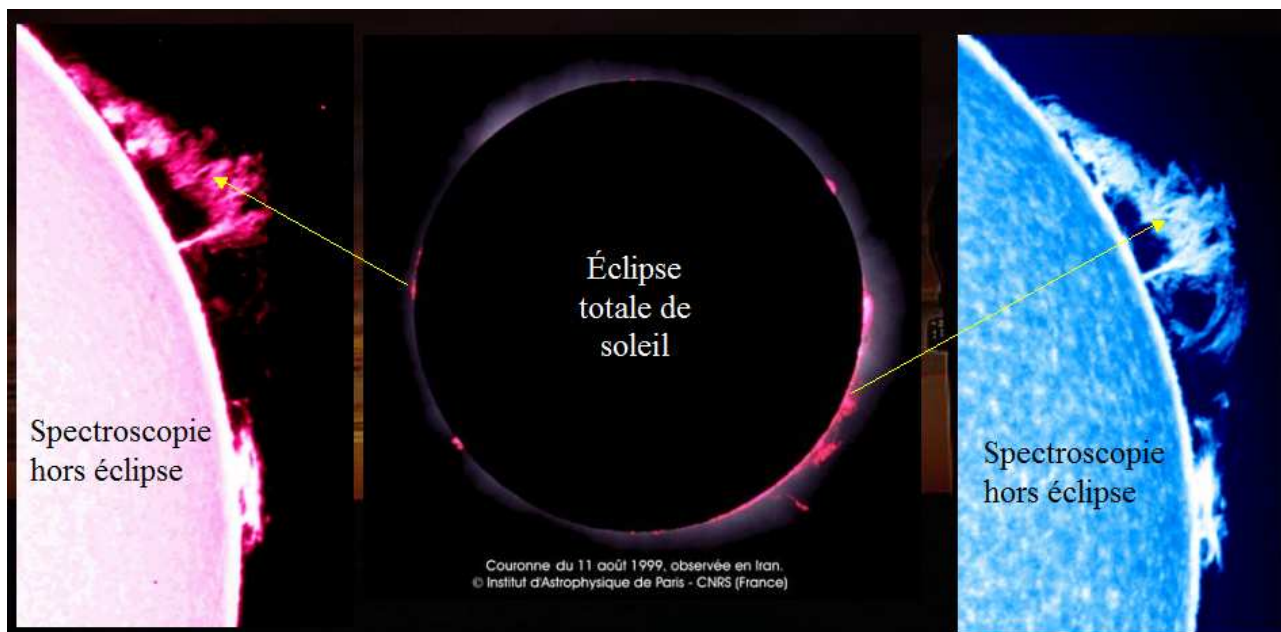
Figure 18 : Janssen et Lockyer démontrent la possibilité d'observer les protubérances hors éclipses grâce à la spectroscopie (clichés Obs. Paris, sauf l'image centrale qui a été obtenue par une équipe de l'Institut d'Astrophysique du CNRS en 1999). Les protubérances sont depuis observées quotidiennement à Meudon grâce à ces techniques.
