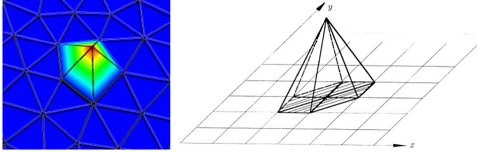
FIG. 11.4 – Base de V_h : exemple de fonction de base globale \varphi_i sur un maillage avec des éléments triangulaires P_1 .
