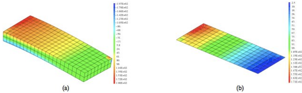
FIG. 10.2 – Contrainte axiale sur la peau supérieure : (a) modèle 3D, (b) modèle ZD.
