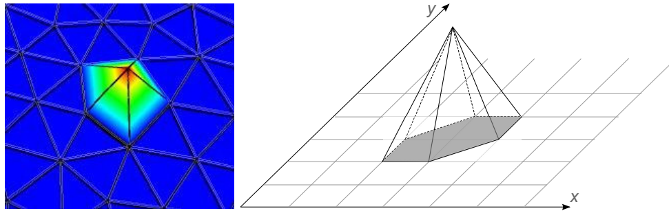
Figure 12.4: Base de V_h : exemple de fonction de base globale \varphi_i sur un maillage avec des éléments triangulaires P_1 .
