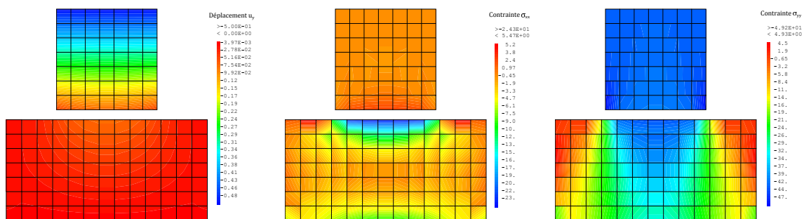
Figure 17.6: a) déplacement u_y b) \sigma_{xx} et c) \sigma_{yy}
