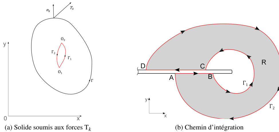
Figure 18.4: Calcul de l'intégrale J
