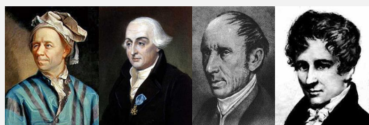
Euler Lagrange Cauchy Abel
