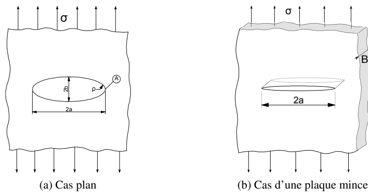
Figure 18.1: Concentration de contraintes autour d'une fissure
