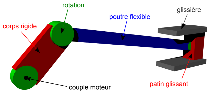
Figure 19.1: Exemple de système multi-corps
