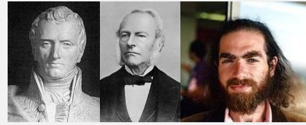
Navier Stokes Perelman
