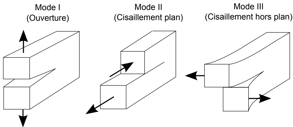
Figure 18.3: Modes de chargement d'une fissure
