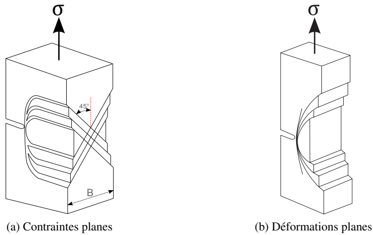
Figure 18.5: Zones de plastification d'une éprouvette entaillée en traction
