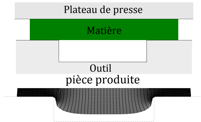
Figure 17.7: Thermocompression : a) problème, b) forme de la pièce après production
