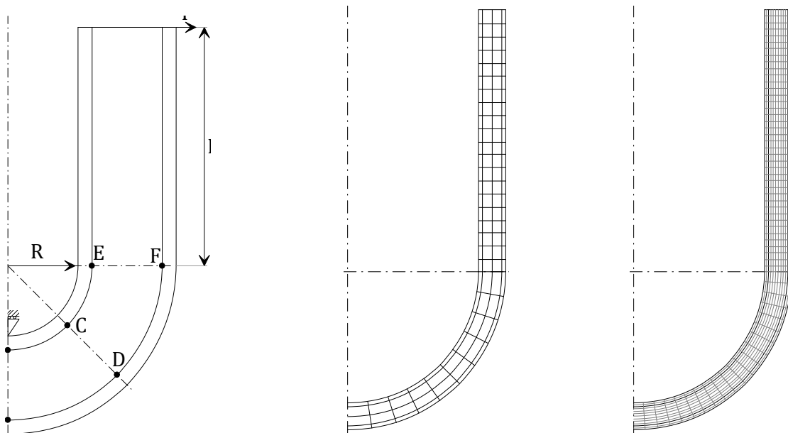
Figure 13.1: a) Géométrie de la poutre en U, b) le maillage utilisé pour le calcul (test de la méthode Reissner local), c) maillage permettant d'obtenir la « solution de référence » puisque'il n'y a pas de solution analytique
