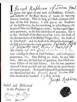
Raphson
