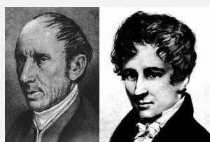
Cauchy Abel
