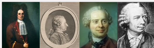
Riccati
