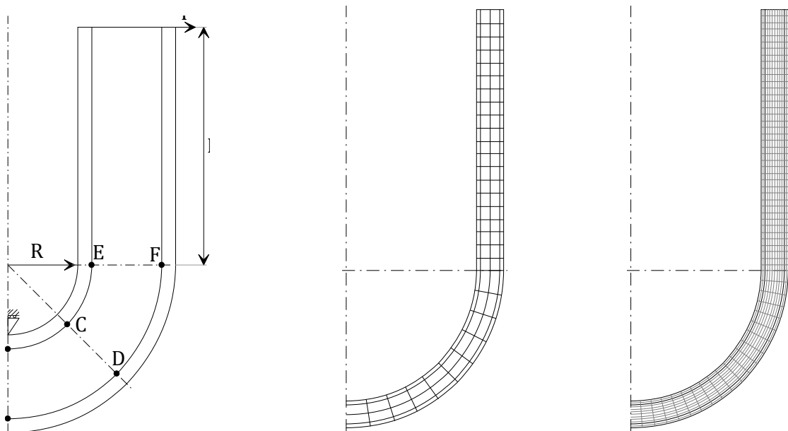
FIGURE 13.1: a) Géométrie de la poutre en U, b) le maillage utilisé pour le calcul (test de la méthode Reissner local, c) maillage permettant d'obtenir la « solution de référence » puisqu'il n'y a pas de solution analytique
