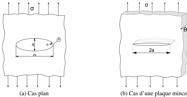
FIGURE 19.1: Concentration de contraintes autour d'une fissure
