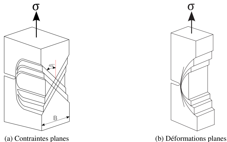
FIGURE 19.5: Zones de plastification d'une éprouvette entaillée en traction
