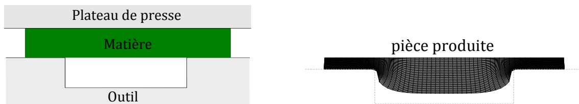
FIGURE 18.7: Thermocompression : a) problème, b) forme de la pièce après production
