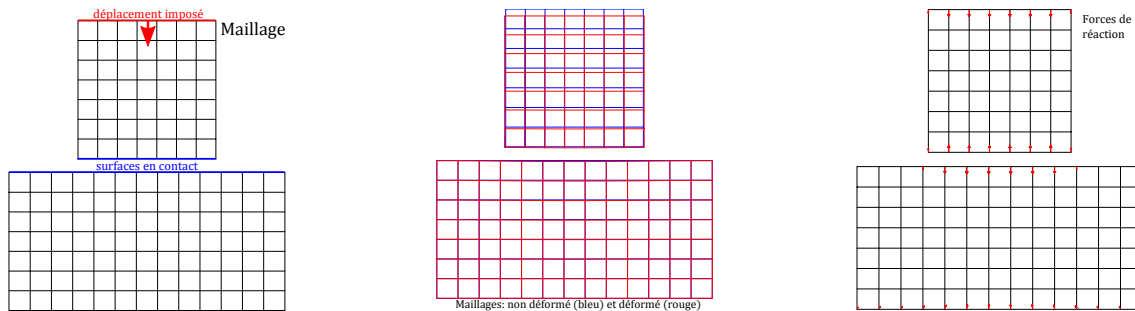
FIGURE 18.5: a) maillage, b) déformée c) forces de réaction
