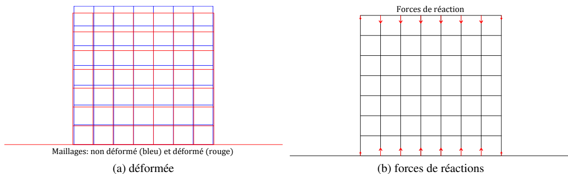
FIGURE 18.4: Premiers résultats sur le contact
