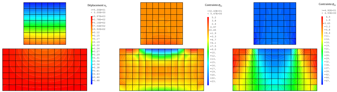
FIGURE 18.6: a) déplacement u_y b) \sigma_{xx} et c) \sigma_{yy}
