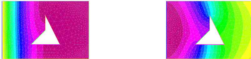
FIGURE 18.15: \Re(p) et \Im(p) à 50 Hz avec un obstacle et 2% d'amortissement
