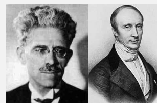
Fréchet
