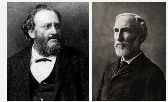
du Bois-Reymond
