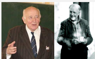
Kurzweil
