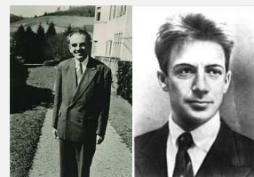
Leray
