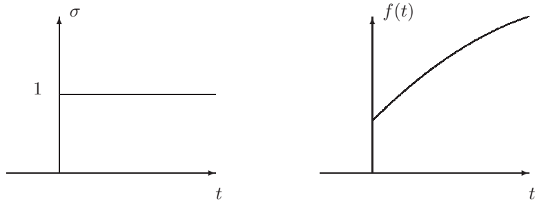
FIG. 15 – Fonction fluage.
