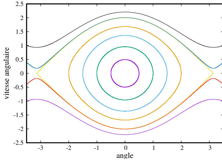
Figure 23: Portrait des phases du pendule. Les trajectoires sont parcourues dans le sens des aiguilles d'une montre. Plusieurs trajectoires fermées (5) avec -\theta_0 < \theta < \theta_0 (et \theta_0 < \pi ) sont représentées en correspondance avec 5 valeurs d'énergie différentes E < 2 . La trajectoire fermée permettant l'amplitude la plus large avec \theta_0 proche de \pi est obtenue pour une énergie E = 2 - \epsilon (avec \epsilon \ll 1 ). Des solutions passantes, obtenues pour E > 2 , sont aussi obtenues, avec 2 trajectoires de type rotation (dans un sens donné dans l'espace physique) au dessus de l'axe des abscisses, et 2 autres trajectoires symétriques de type rotation en sens inverse en dessous de l'axe.
