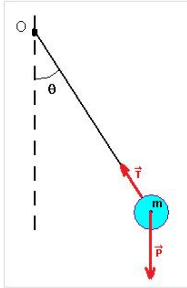
Figure 22: Le pendule est constitué d'une masse m suspendue au bout d'un fil inextensible de longueur l et oscillant dans le champ de pesanteur d'intensité g . La masse supposée ponctuelle est soumise à son poids d'intensité P = mg et à la tension du fil d'intensité T .
