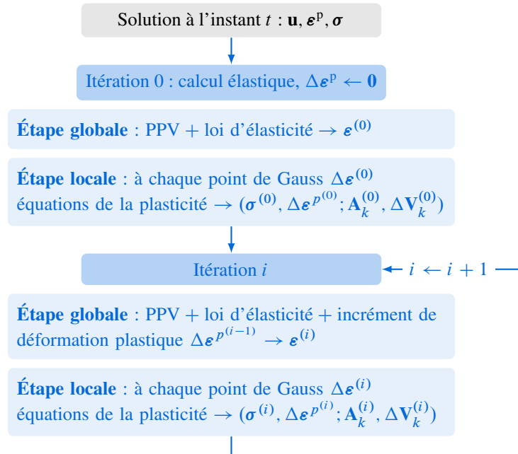
Figure 4.1 – Résolution du problème élastoplastique par la méthode des éléments finis
