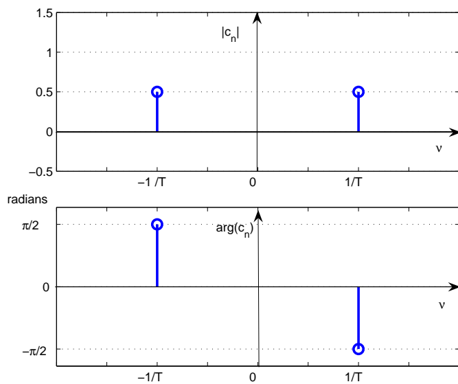
FIG. 2.4 – Représentation des coefficients c_n de la série de Fourier
